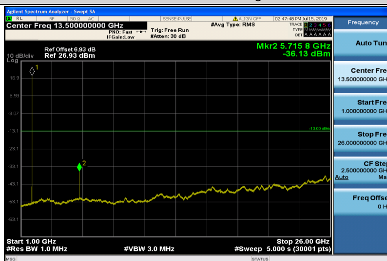
Band2-5MHz-QPSK-19175-1RB#0-Range2:1000~26000MHz
