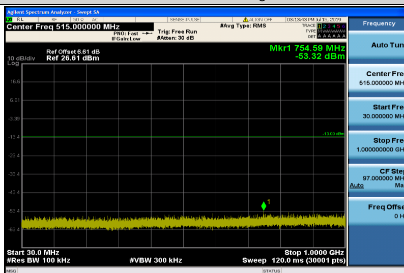
Band2-20MHz-QPSK-18900-1RB#0-Range1:30~1000MHz
