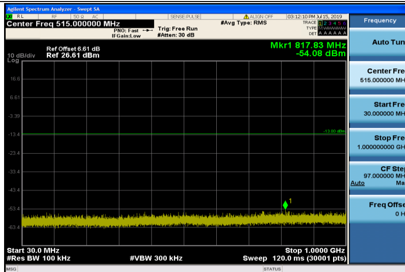
Band2-20MHz-QPSK-18700-1RB#0-Range1:30~1000MHz
