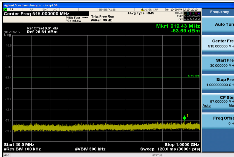
Band4-10MHz-QPSK-20000-1RB#0-Range1:30~1000MHz
