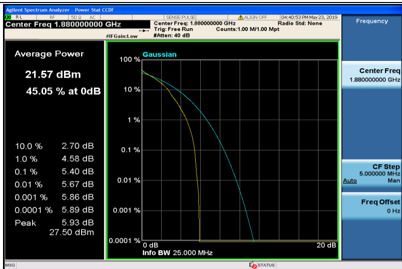
Band2-5MHz-QPSK-18900-1RB#0
