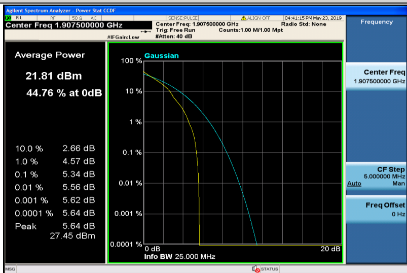
Band2-5MHz-QPSK-19175-1RB#0
