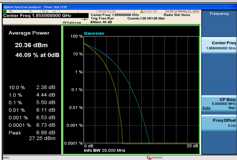
Band2-10MHz-QPSK-18650-50RB#0
