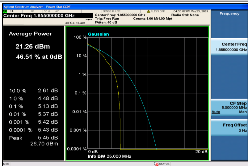
Band2-10MHz-QPSK-18650-1RB#0
