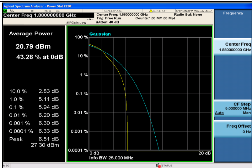
Band2-5MHz-16QAM-18900-1RB#0
