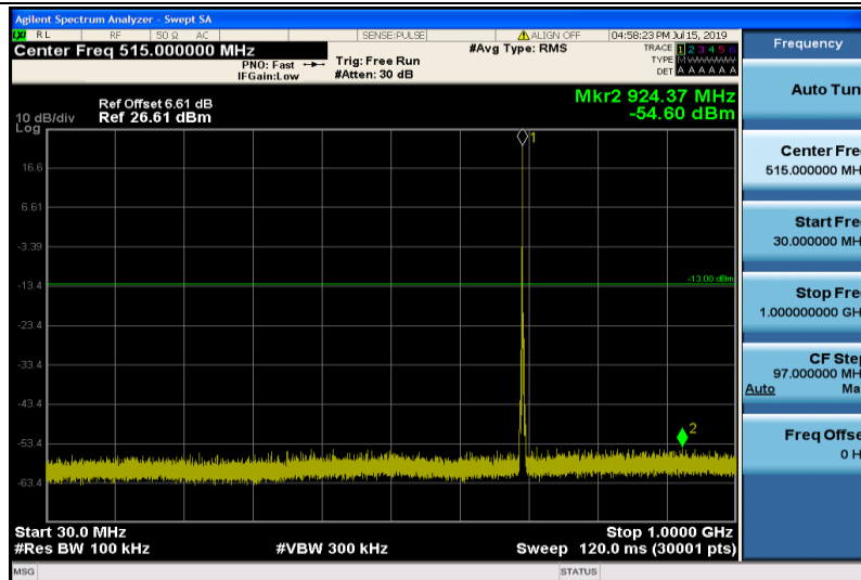
Band12-1.4MHz-QPSK-23017-1RB#0-Range1:30~1000MHz
