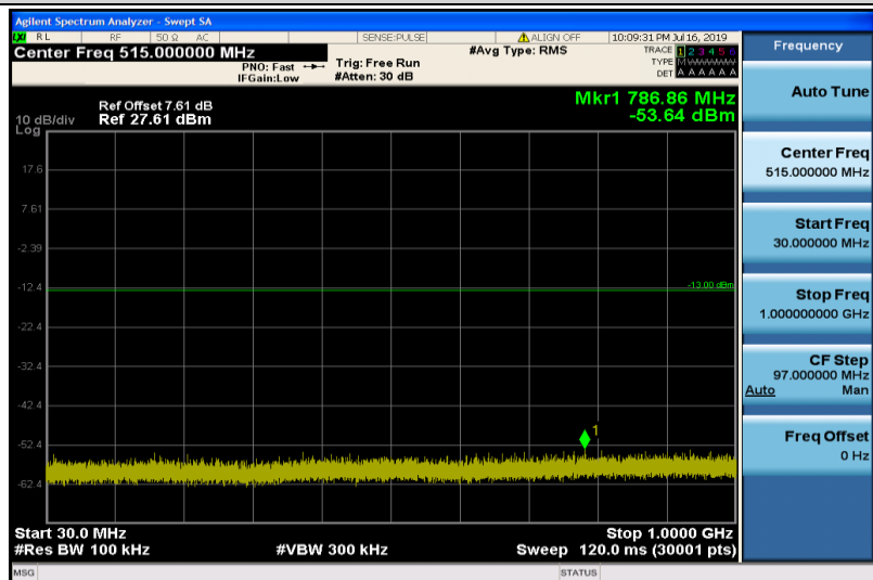
Band25-20MHz-QPSK-26590-1RB#0-30~1000MHz
