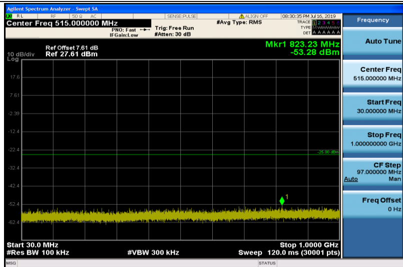
Band41-10MHz-QPSK-40290-1RB#0-30~1000MHz
