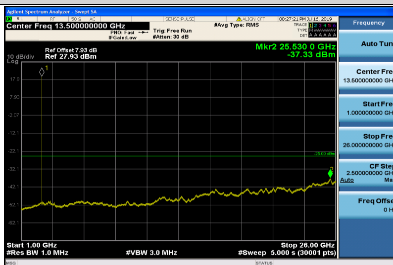
Band41-5MHz-QPSK-41215-1RB#0-1000~26000MHz
