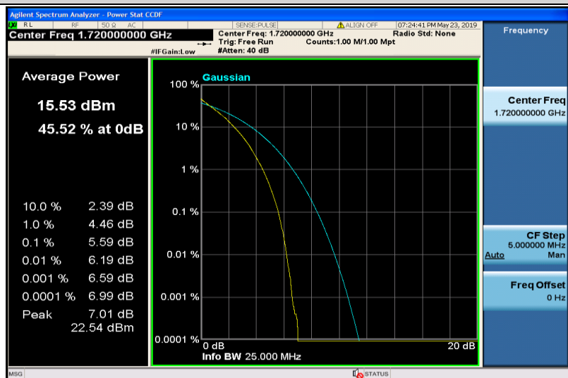
Band4-20MHz-QPSK-20050-100RB#0
