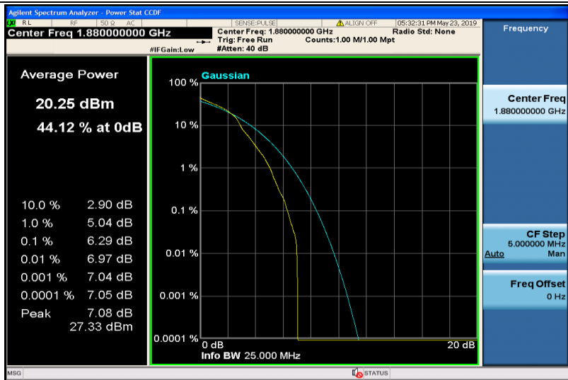
Band2-20MHz-16QAM-18900-1RB#0
