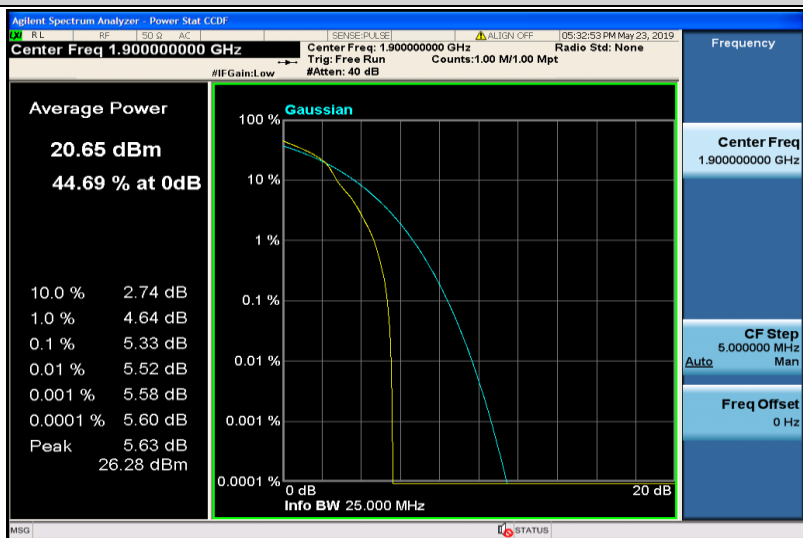
Band2-20MHz-16QAM-19100-1RB#0
