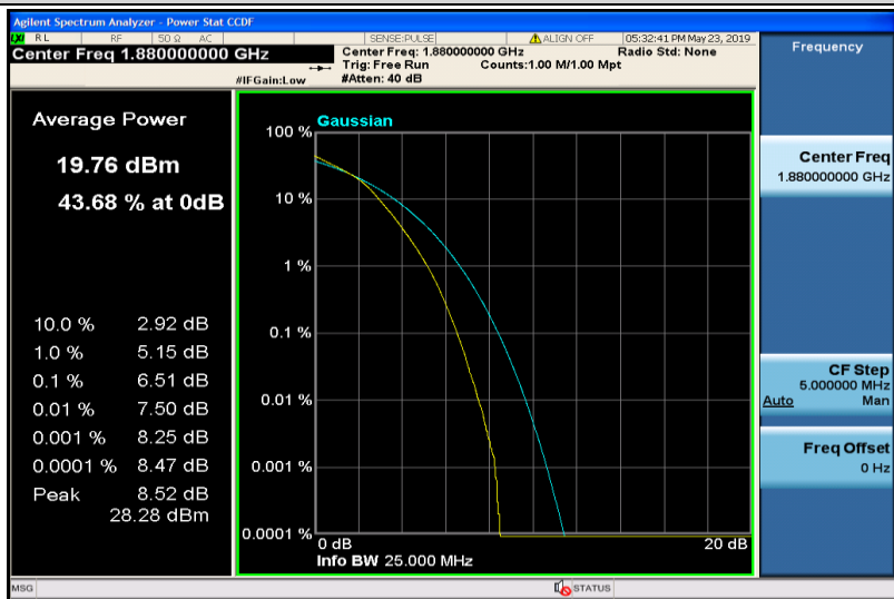
Band2-20MHz-16QAM-18900-100RB#0
