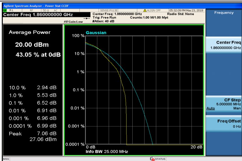
Band2-20MHz-16QAM-18700-1RB#0
