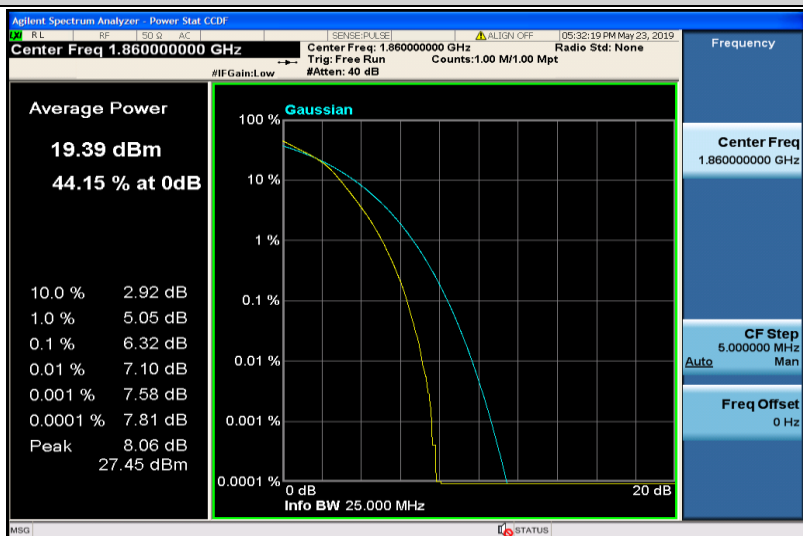
Band2-20MHz-16QAM-18700-100RB#0
