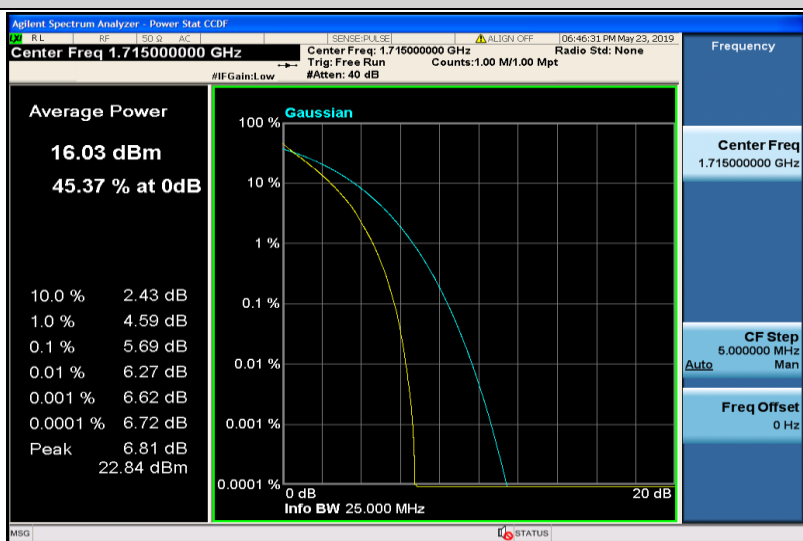
Band4-10MHz-QPSK-20000-50RB#0
