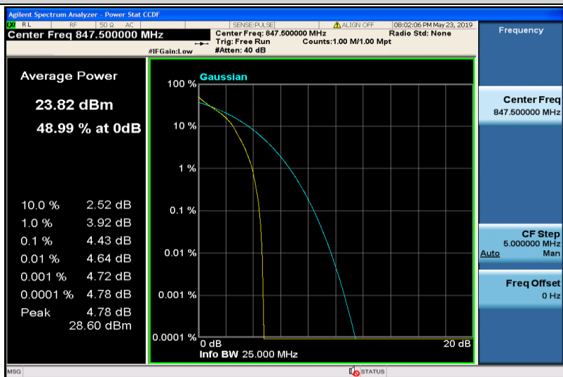
Band5-3MHz-QPSK-20635-1RB#0
