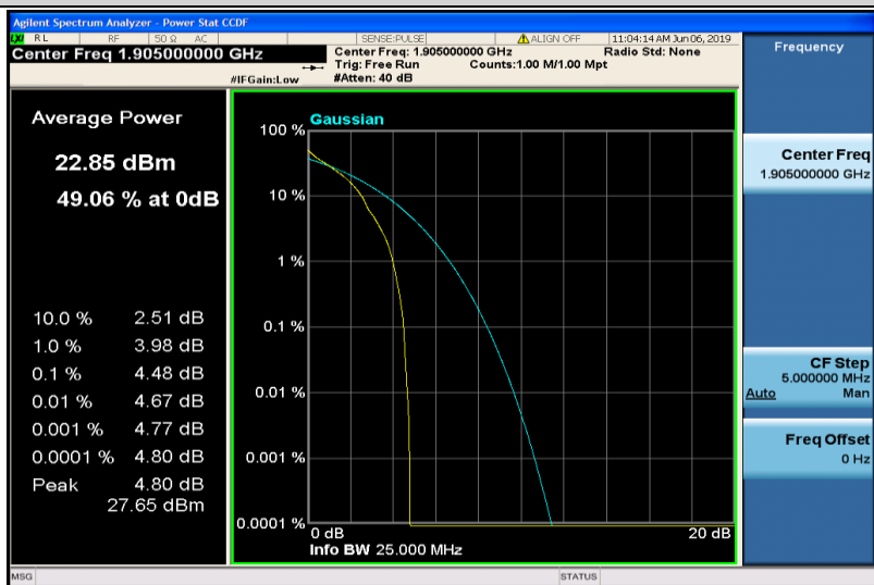
Band25-20MHz-QPSK-26590-1RB#0
