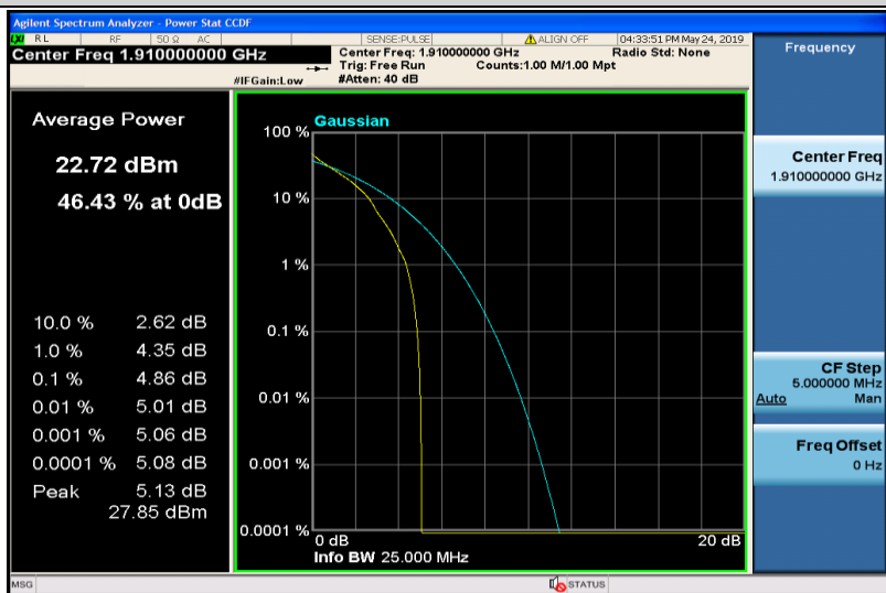
Band25-10MHz-QPSK-26640-1RB#0
