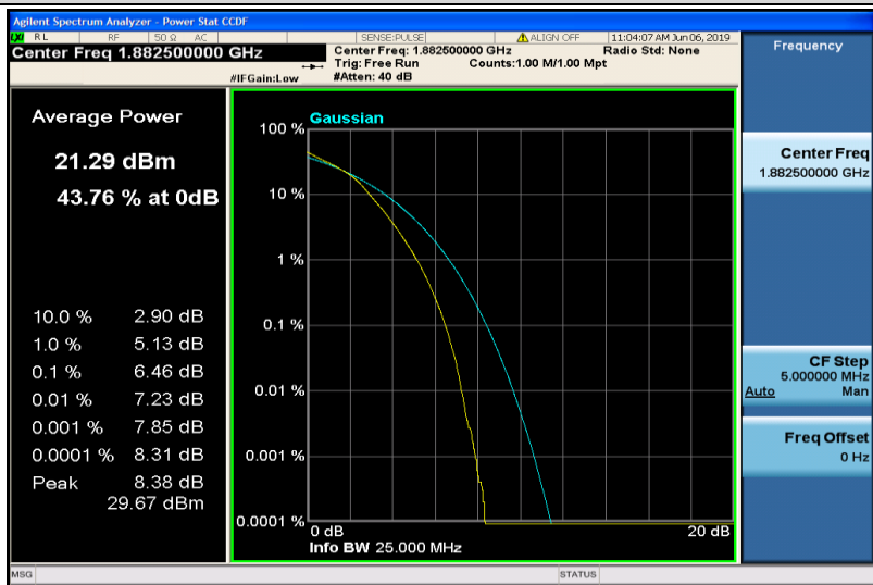
Band25-20MHz-16QAM-26365-100RB#0
