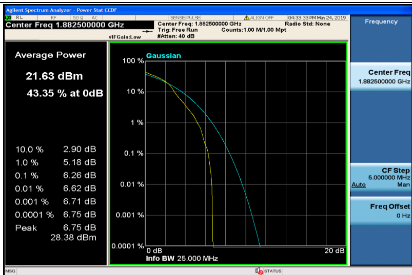
Band25-10MHz-16QAM-26365-1RB#0
