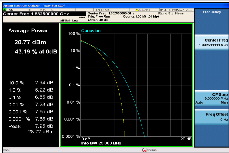
Band25-10MHz-16QAM-26365-50RB#0
