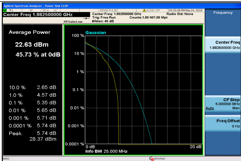
Band25-10MHz-QPSK-26365-1RB#0
