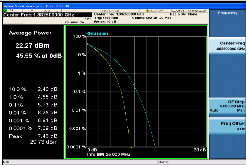
Band25-20MHz-QPSK-26365-100RB#0
