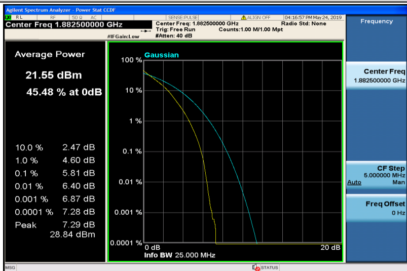
Band25-5MHz-QPSK-26365-25RB#0
