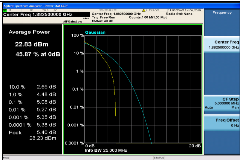
Band25-20MHz-QPSK-26365-1RB#0
