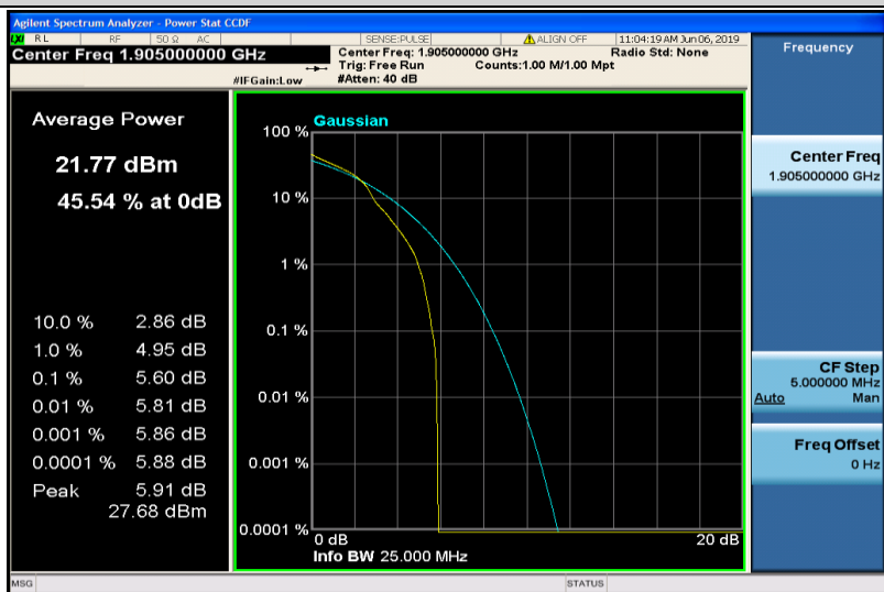
Band25-20MHz-16QAM-26590-1RB#0
