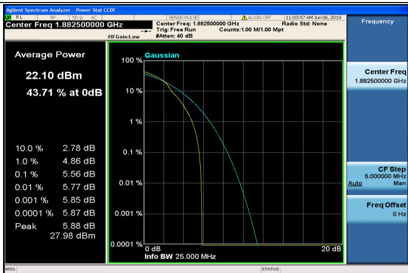
Band25-20MHz-16QAM-26365-1RB#0
