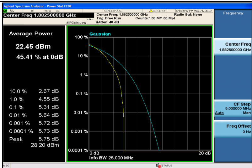
Band25-5MHz-QPSK-26365-1RB#0
