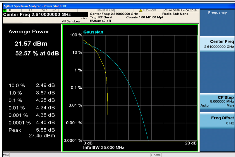
Band38-20MHz-QPSK-38150-1RB#0
