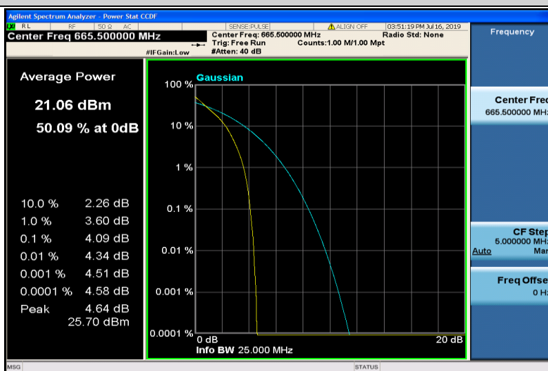
Band71-5MHz-QPSK-133147-25RB#0
