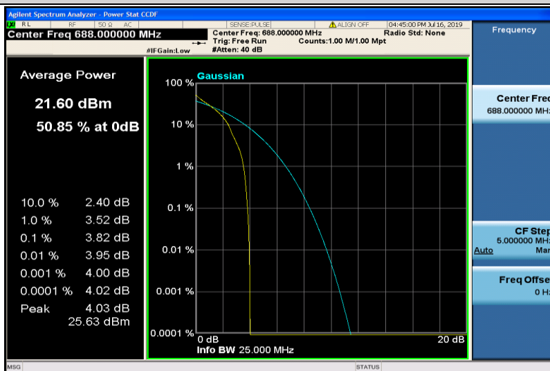
Band71-20MHz-QPSK-133372-1RB#0
