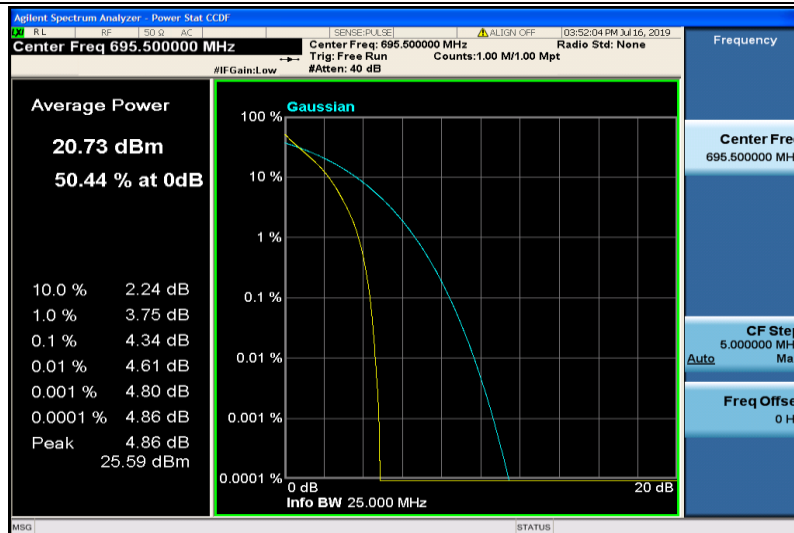
Band71-5MHz-QPSK-133447-25RB#0
