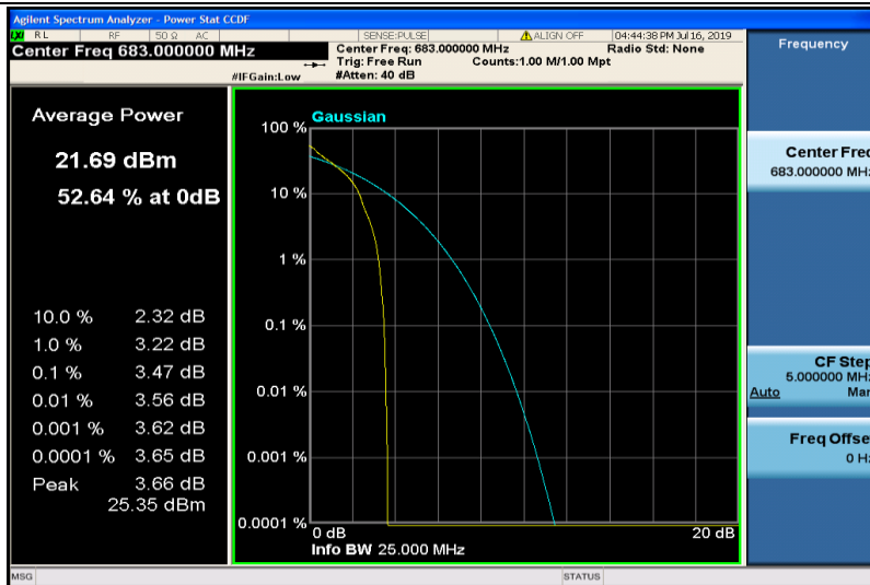
Band71-20MHz-QPSK-133322-1RB#0
