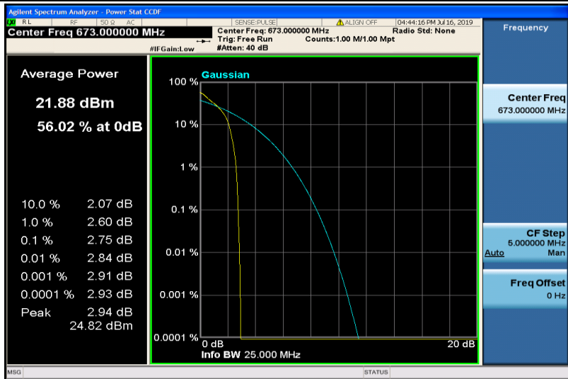
Band71-20MHz-QPSK-133222-1RB#0
