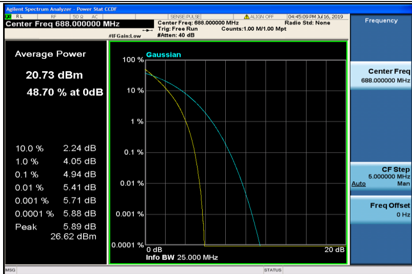
Band71-20MHz-QPSK-133372-100RB#0
