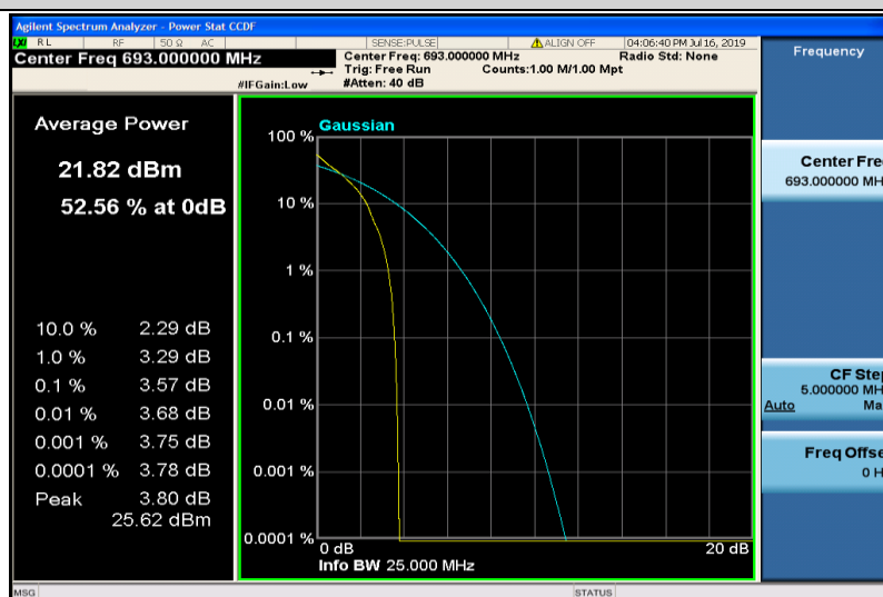
Band71-10MHz-QPSK-133422-1RB#0
