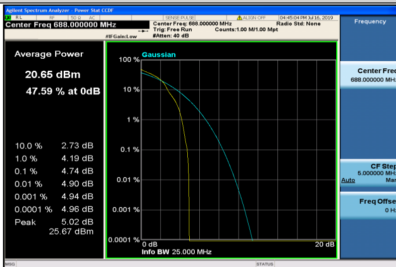
Band71-20MHz-16QAM-133372-1RB#0
