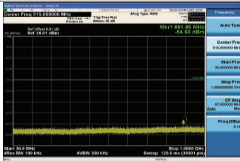
Band4-1.4MHz-QPSK-20393-1RB#0-Range1:30~1000MHz
