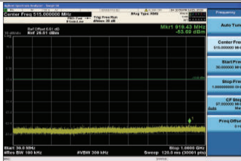
Band4-10MHz-QPSK-20000-1RB#0-Range1:30~1000MHz
