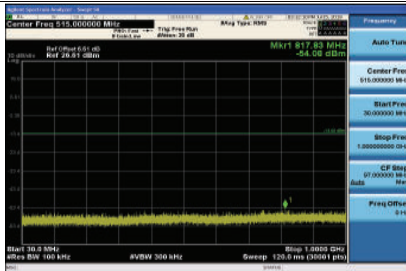
Band2-20MHz-QPSK-18700-1RB#0-Range1:30~1000MHz
