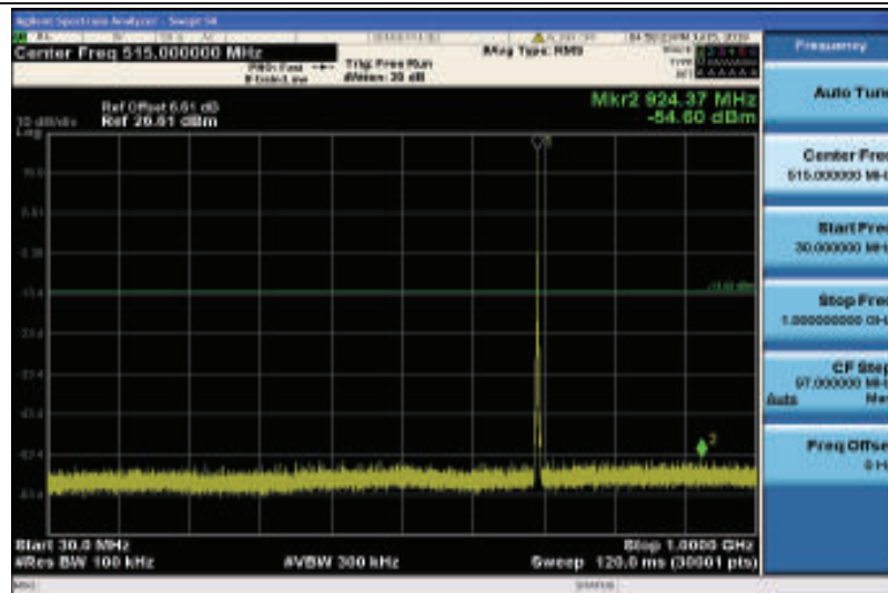
Band12-1.4MHz-QPSK-23017-1RB#0-Range1:30~1000MHz
