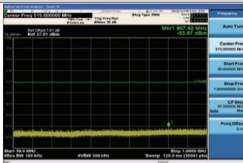
Band25-1.4MHz-QPSK-26365-1RB#0-30~1000MHz
