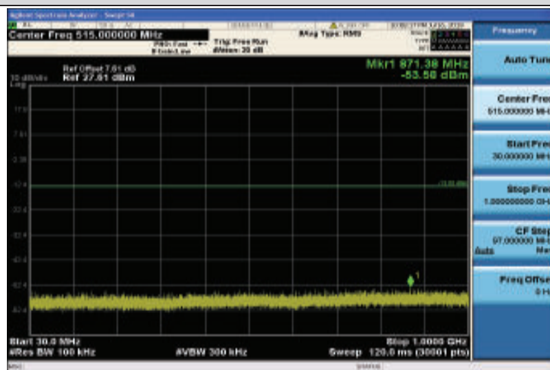
Band25-20MHz-QPSK-26365-1RB#0-30~1000MHz
