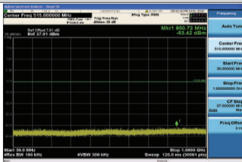
Band25-10MHz-QPSK-26365-1RB#0-30~1000MHz
