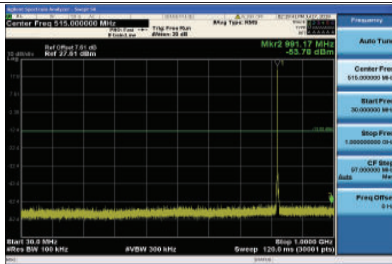
Band26-1.4MHz-QPSK-26797-1RB#0-30~1000MHz
