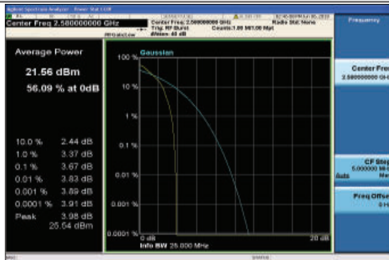
Band38-20MHz-QPSK-37850-1RB#0
