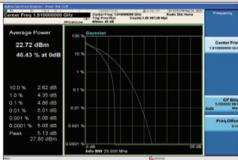
Band25-10MHz-QPSK-26640-1RB#0
