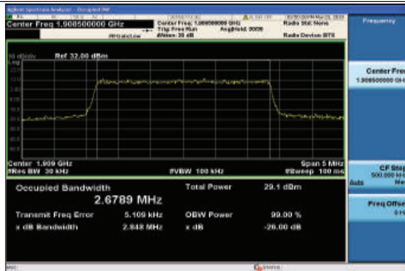
Band2-3MHz-QPSK-19185-15RB#0-2.6789
