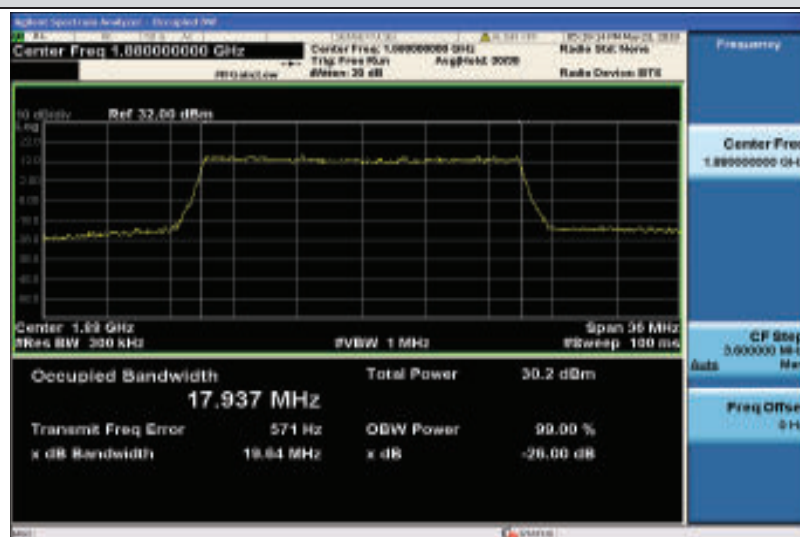
Band2-20MHz-QPSK-18900-100RB#0-17.937
