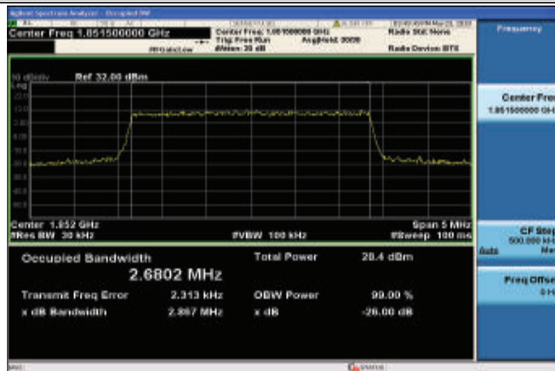
Band2-3MHz-QPSK-18615-15RB#0-2.6802
