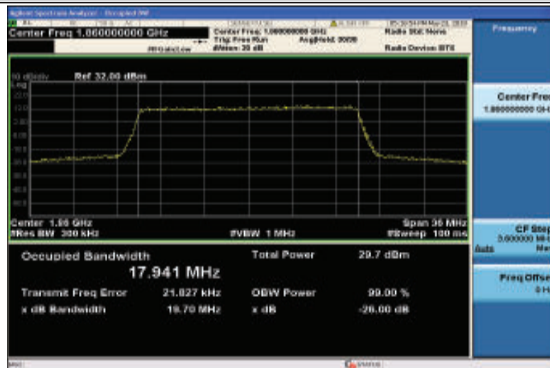
Band2-20MHz-QPSK-18700-100RB#0-17.941
