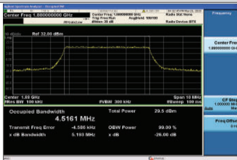
Band2-5MHz-QPSK-18900-25RB#0-4.5161
