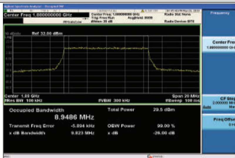
Band2-10MHz-QPSK-18900-50RB#0-8.9486
