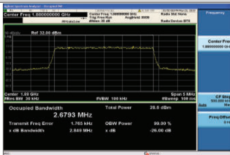
Band2-3MHz-QPSK-18900-15RB#0-2.6793
