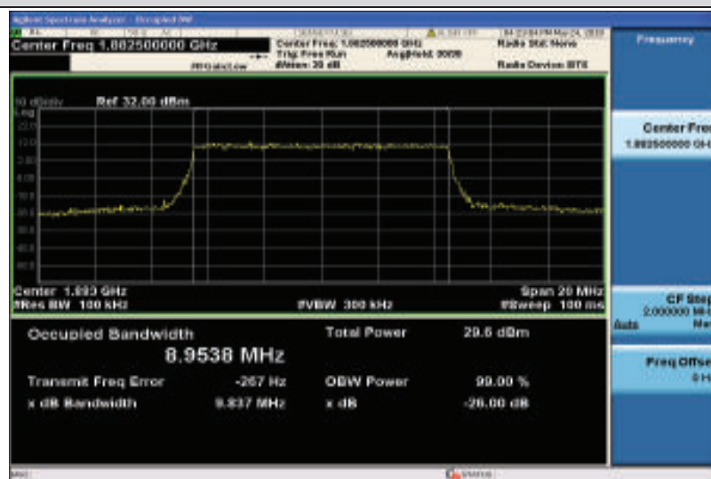
Band25-10MHz-16QAM-26365-50RB#0-8.9538
