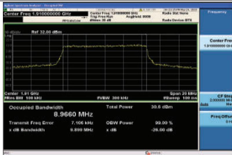
Band25-10MHz-QPSK-26640-50RB#0-8.9660
