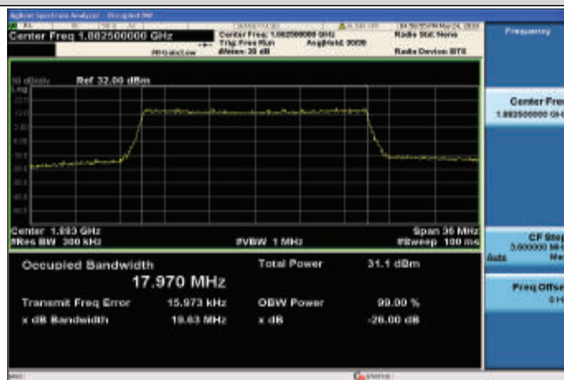
Band25-20MHz-QPSK-26365-100RB#0-17.970
