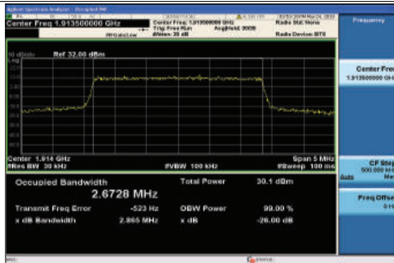
Band25-3MHz-QPSK-26675-15RB#0-2.6728
