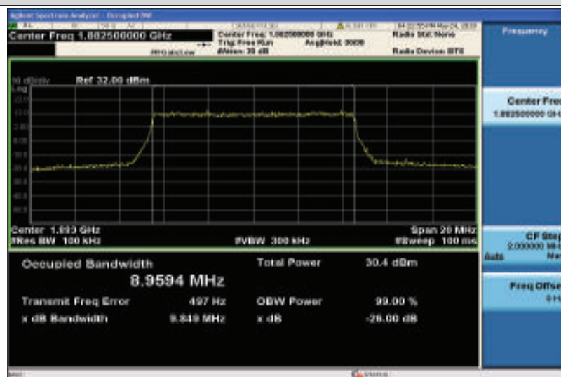
Band25-10MHz-QPSK-26365-50RB#0-8.9594
