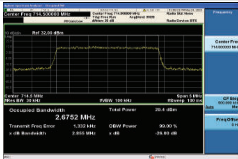
Band12-3MHz-QPSK-23165-15RB#0-2.6752
