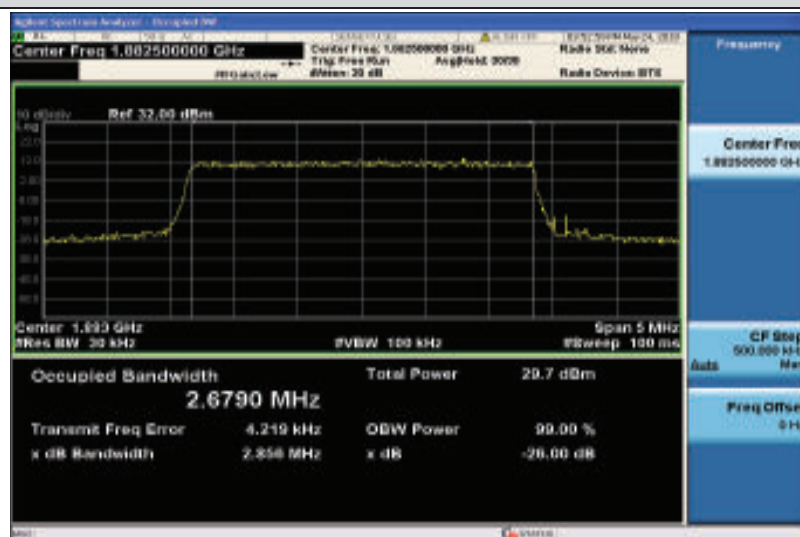
Band25-3MHz-QPSK-26365-15RB#0-2.6790
