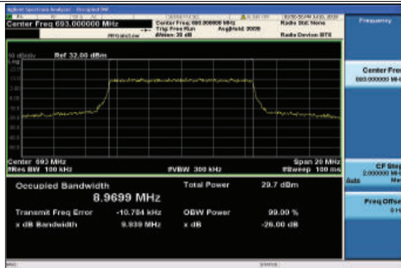
Band71-10MHz-QPSK-133422-50RB#0-8.9699
