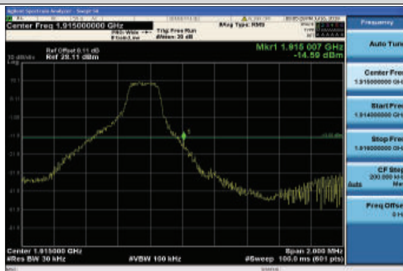
Band25-3MHz-QPSK-26675-1RB#14
