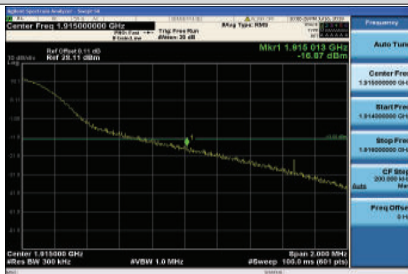
Band25-20MHz-16QAM-26590-1RB#99
