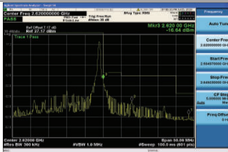
Band38-20MHz-QPSK-38150-1RB#99
