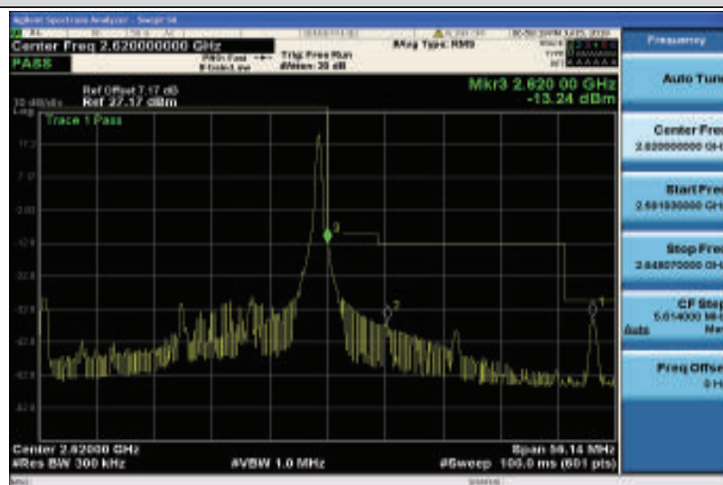
Band38-15MHz-QPSK-38175-1RB#74
