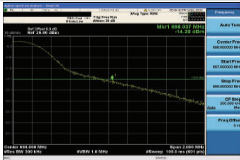
Band71-15MHz-QPSK-133397-1RB#74
