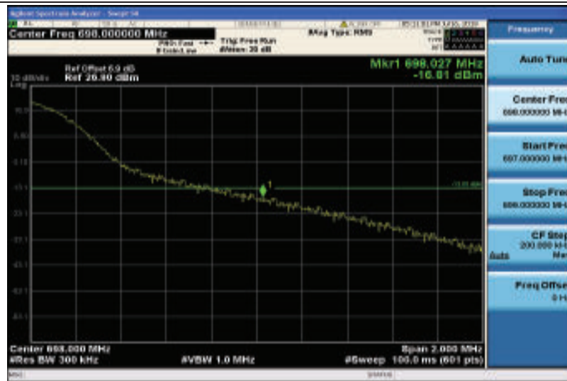
Band71-20MHz-16QAM-133372-1RB#99
