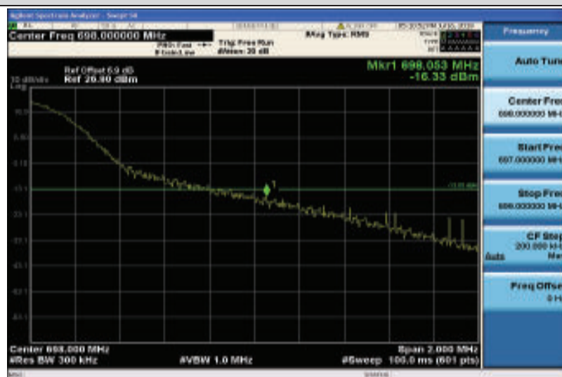
Band71-20MHz-QPSK-133372-1RB#99
