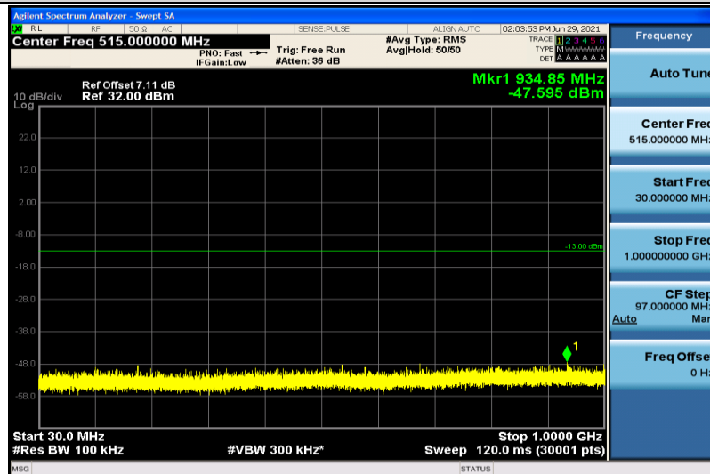
Band4-3MHz-QPSK-20385-1RB#0-30~1000MHz
