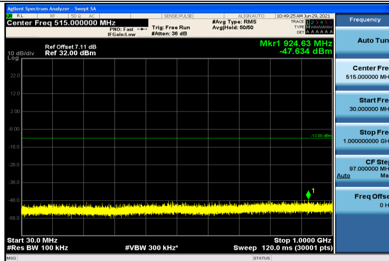
Band2-10MHz-QPSK-19150-1RB#0-30~1000MHz
