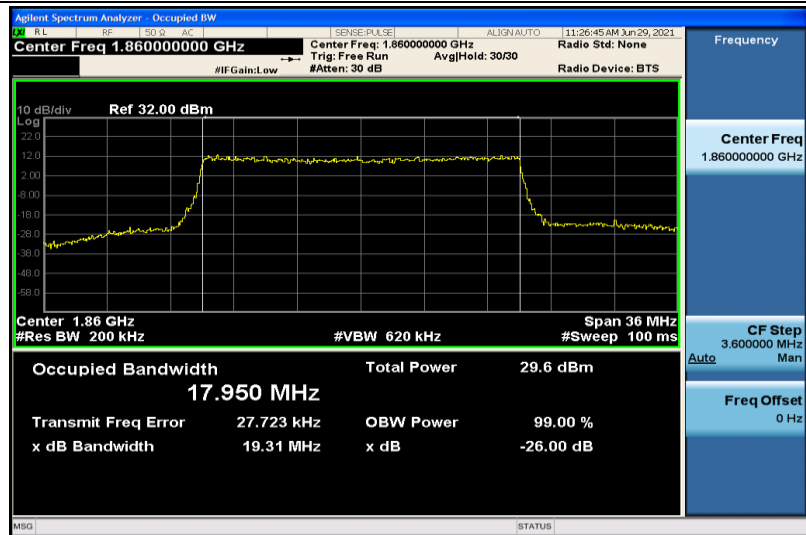
Band2-20MHz-16QAM-18700-100RB#0-17.950
