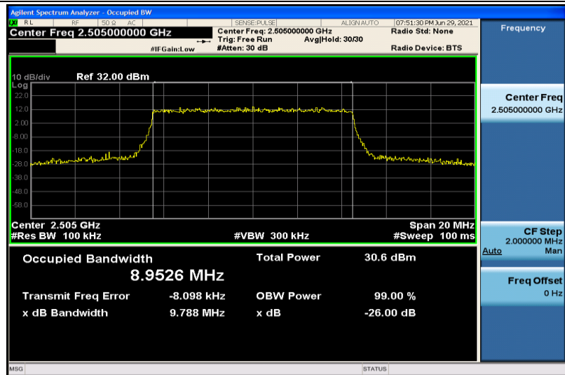
Band7-10MHz-QPSK-20800-50RB#0-8.9526
