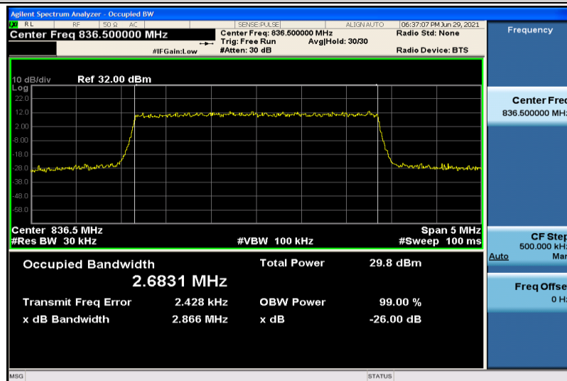
Band5-3MHz-QPSK-20525-15RB#0-2.6831
