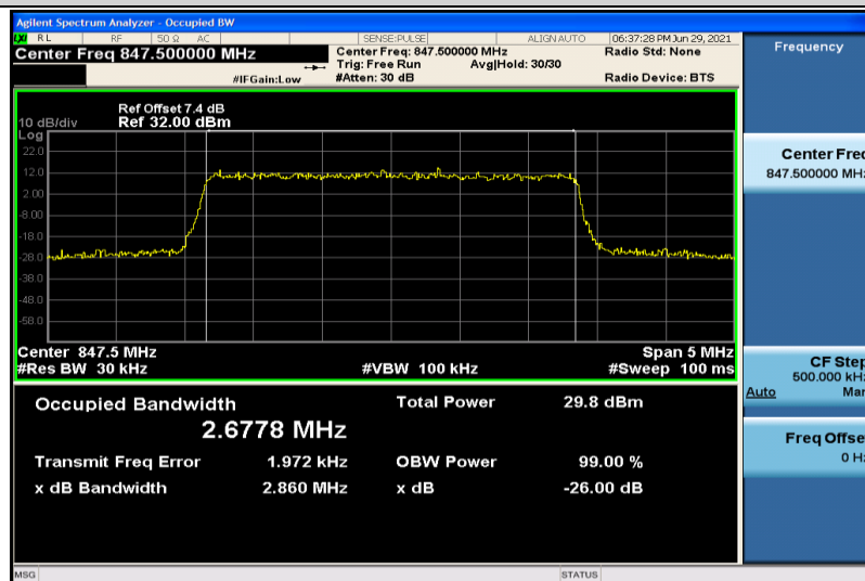
Band5-3MHz-QPSK-20635-15RB#0-2.6778
