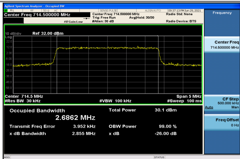
Band12-3MHz-QPSK-23165-15RB#0-2.6862
