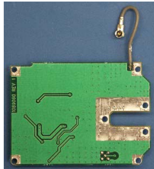
Pre amp Bottom
