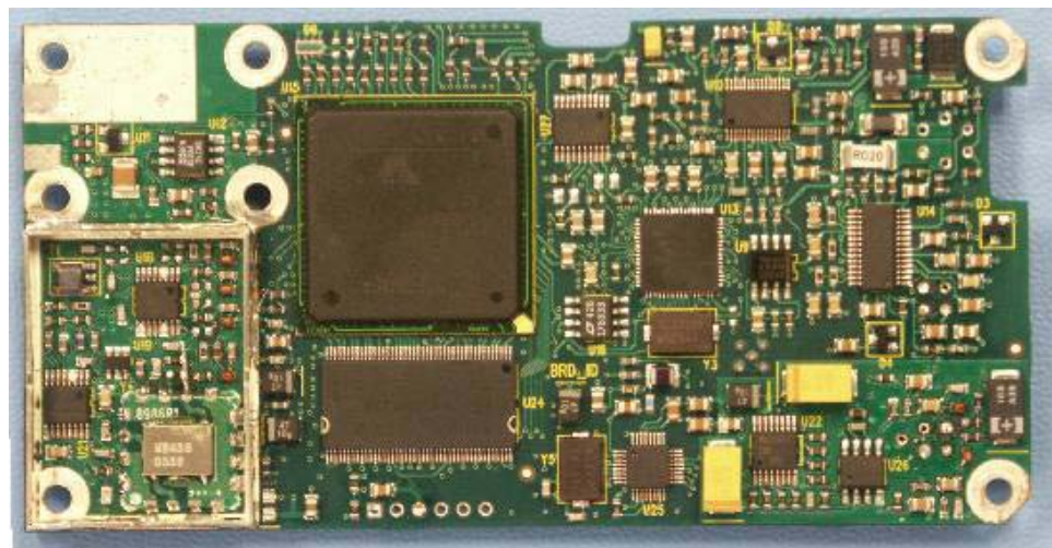
PCB Bottom
