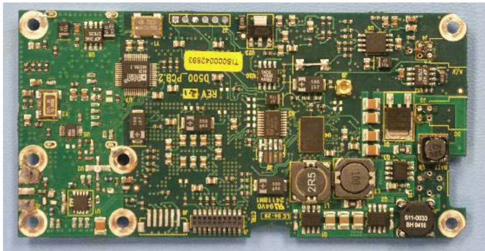
PCB Top
