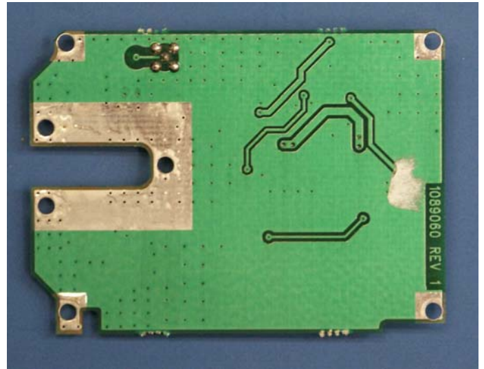
PA Bottom
