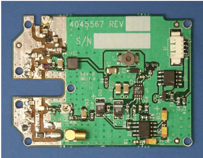
PA Top
