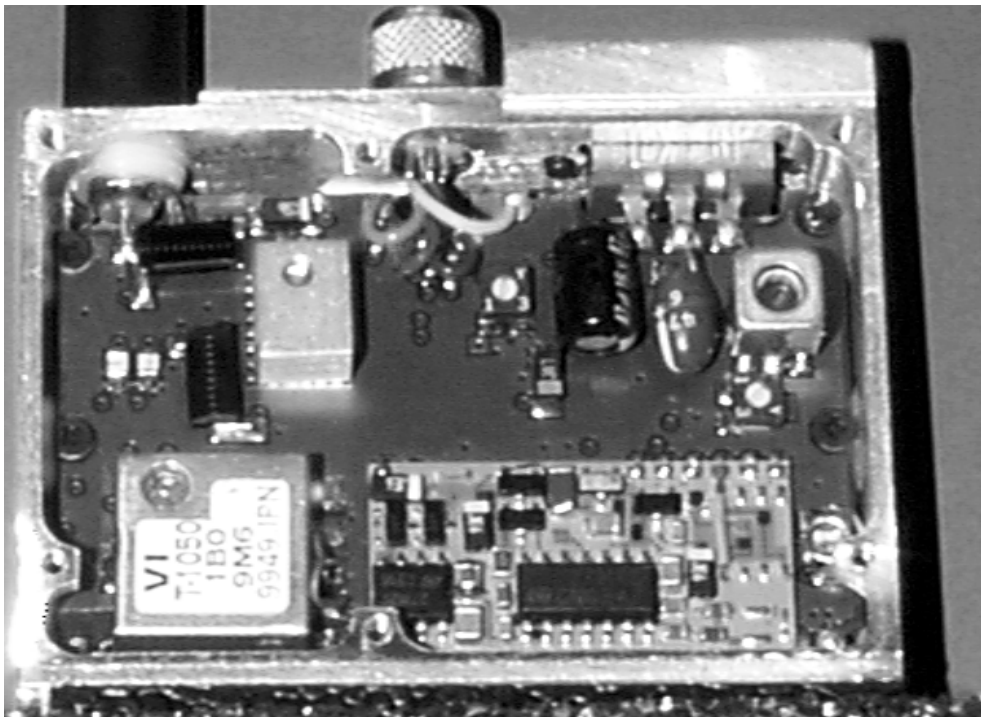
Bottom Side
