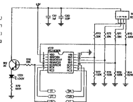
PC16C505 16個CH切換 含透DISPLAY資料輸出 預計使用內部OSC=4MHz
