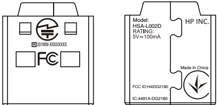
Seal: 2:1
