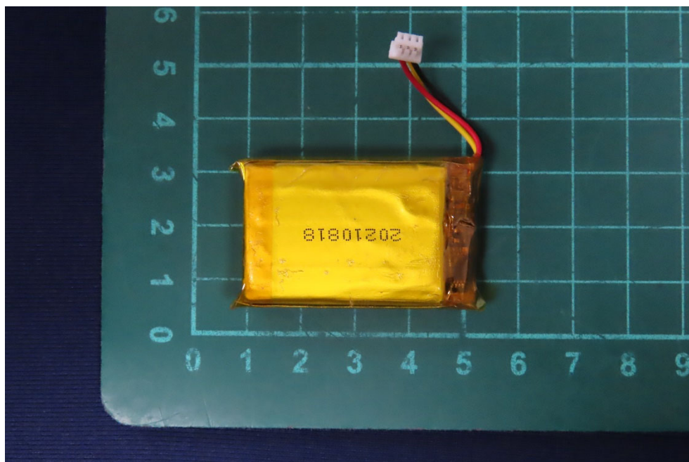
(24) EUT Photo
