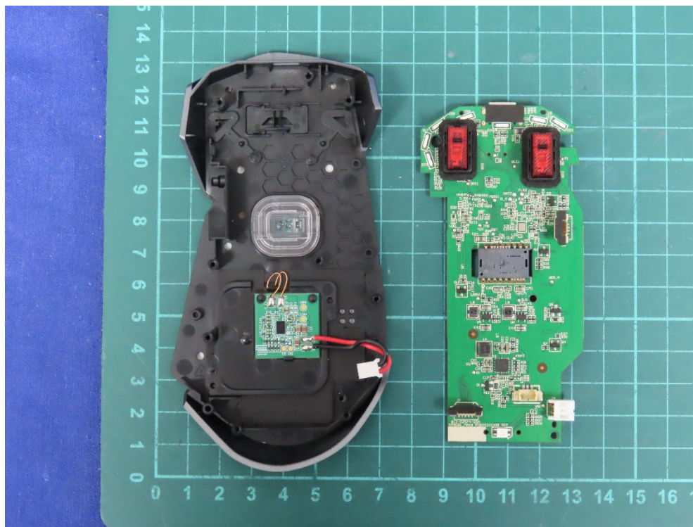
(20) EUT Photo
