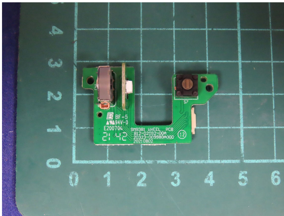
(10) EUT Photo
