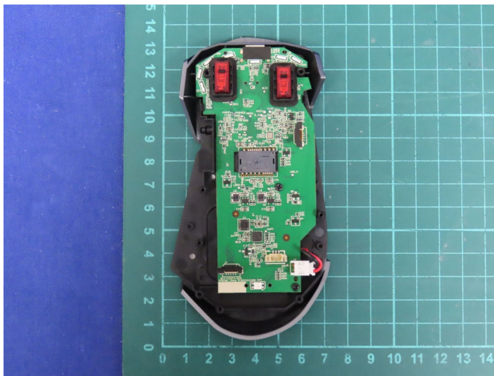
(19) EUT Photo
