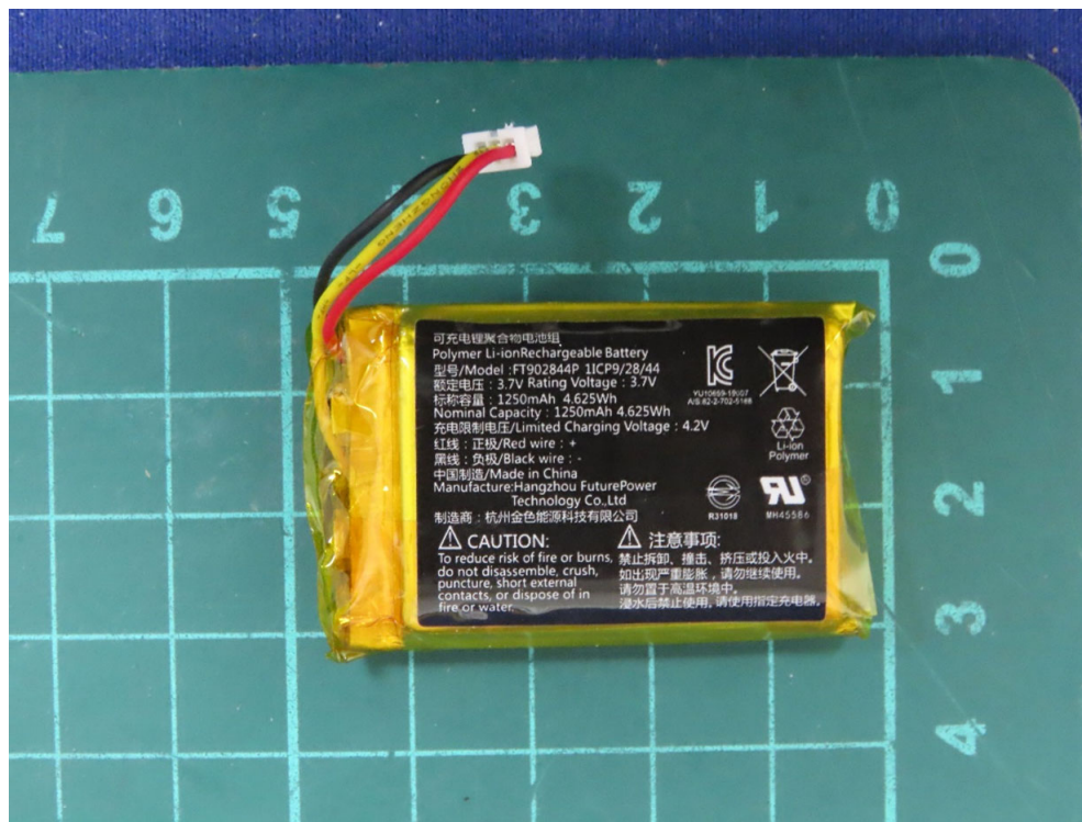
(16) EUT Photo
