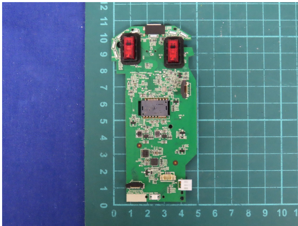
(21) EUT Photo
