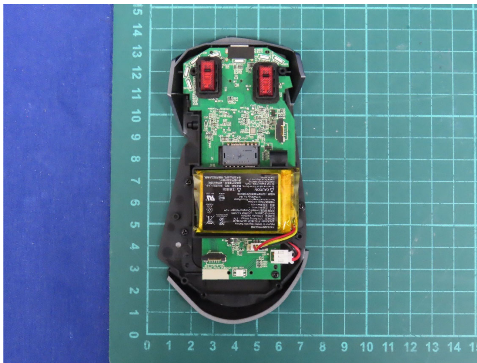
(12) EUT Photo
