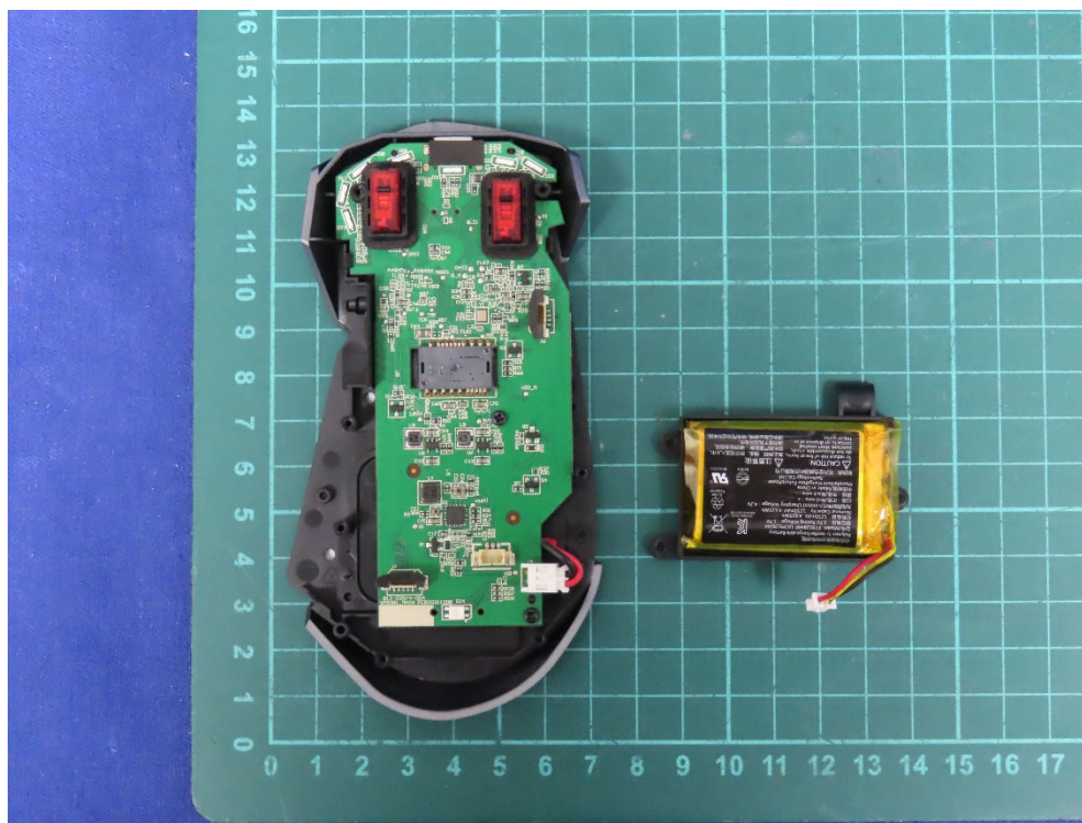
(13) EUT Photo
