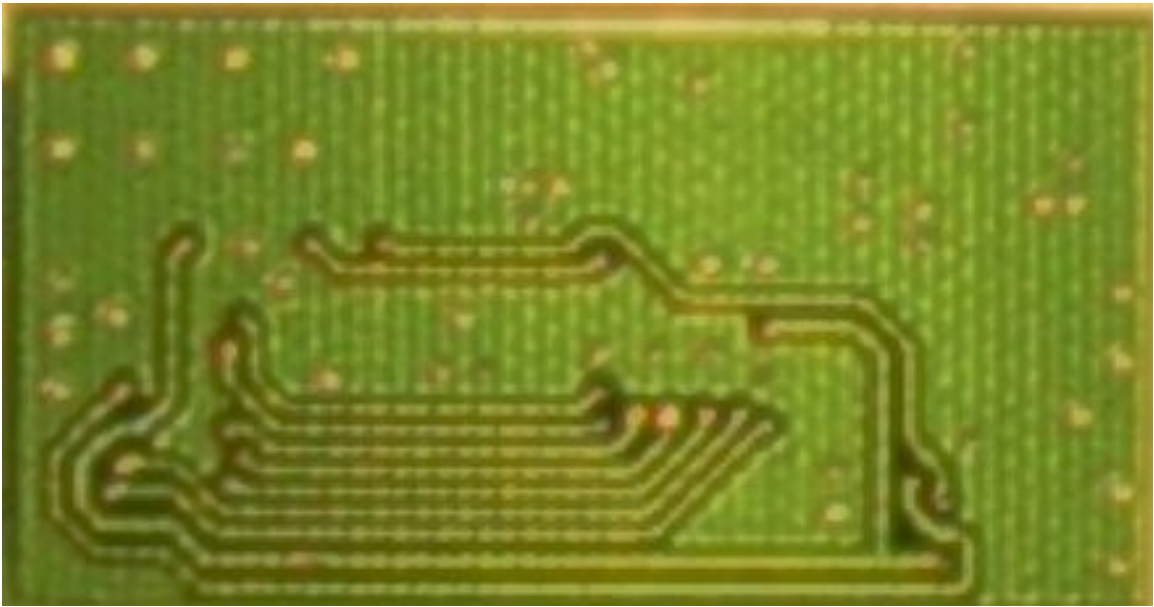
Fig. 6 – CTCSS PCB rear side
