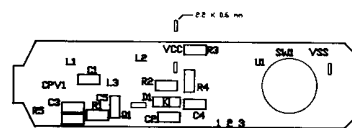
512 Top Overlay
