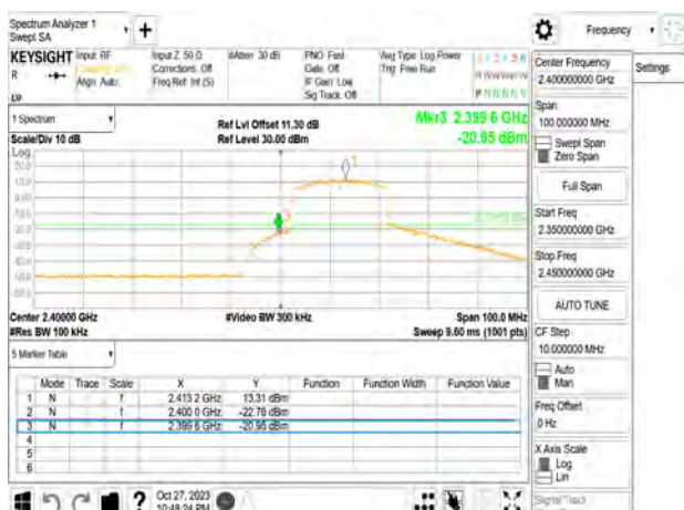
802.11be_20MHz_Chain0_2412MHz
