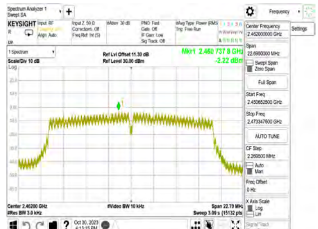
802.11g_20MHz_Chain3_2462MHz
