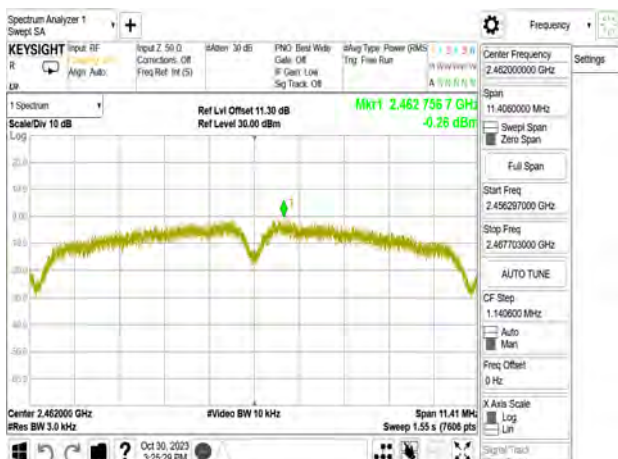
802.11b_20MHz_Chain2_2462MHz
