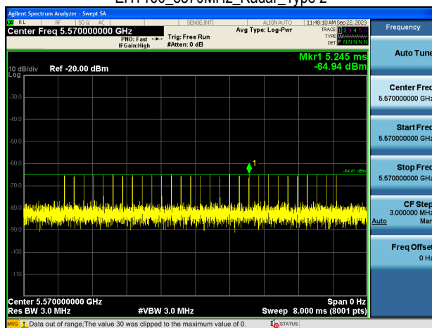
EHT160_5570MHz_Radar_Type 2
