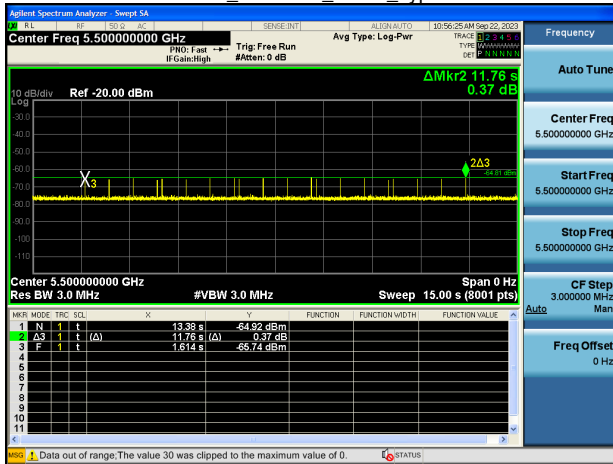
EHT20_5500MHz_Radar_Type 6
