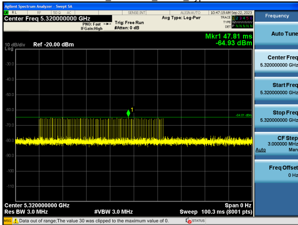
EHT20_5320MHz_Radar_Type 2
