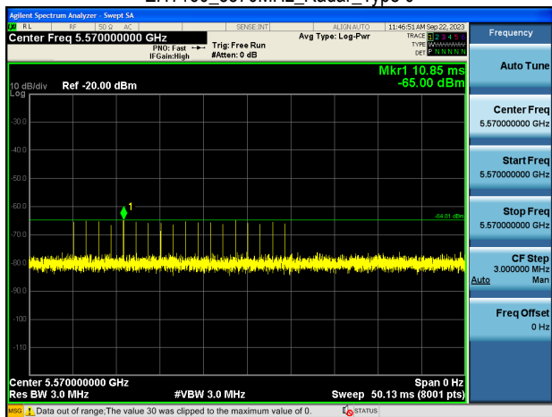
EHT160_5570MHz_Radar_Type 0
