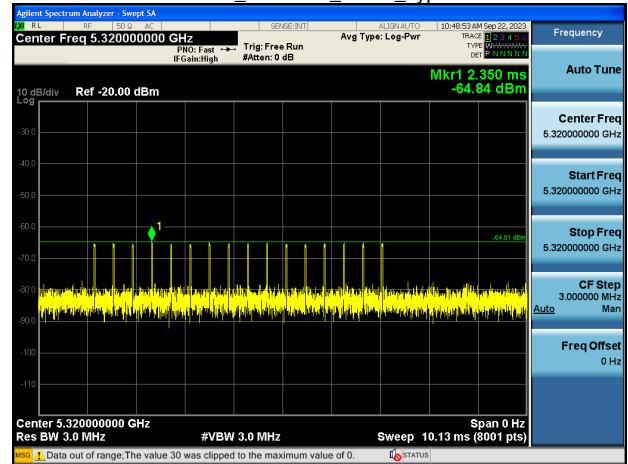
EHT20_5320MHz_Radar_Type 5
