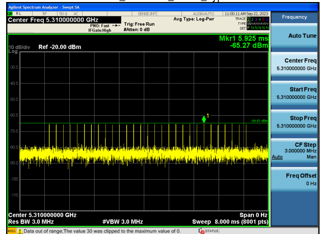
EHT40_5310MHz_Radar_Type 2
