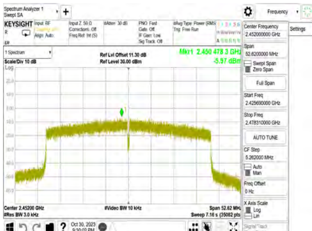
802.11be_40MHz_Chain0_2452MHz
