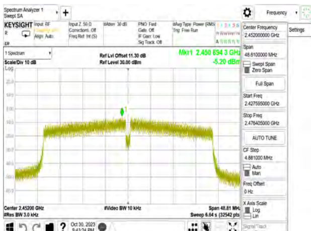
802.11n_40MHz_Chain2_2452MHz
