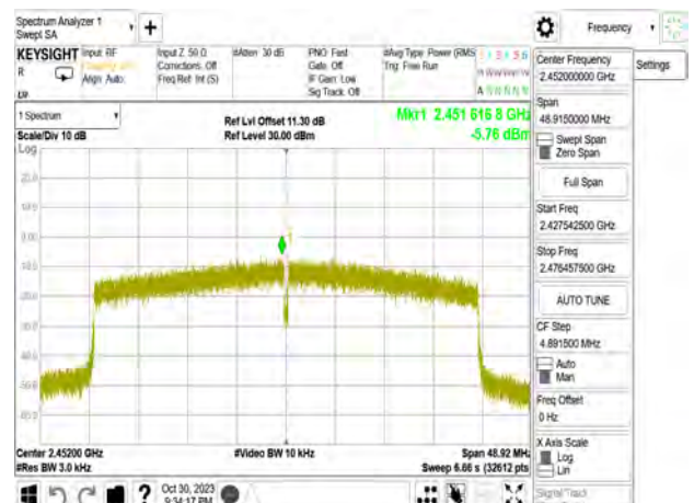
802.11be_40MHz_Chain3_2452MHz
