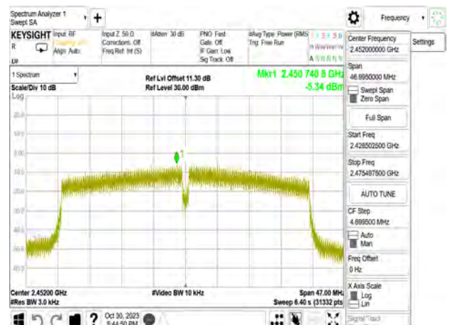
802.11n_40MHz_Chain3_2452MHz
