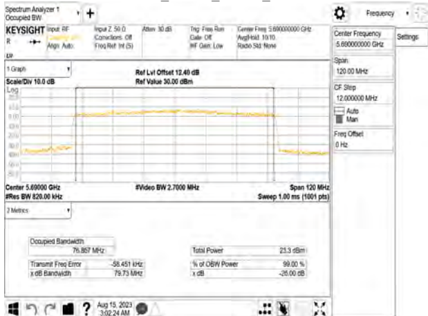
802.11be_80MHz_Chain3_5690MHz
