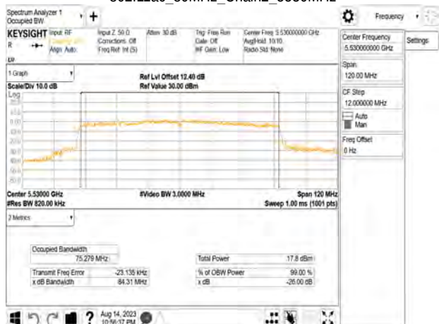
802.11ac_80MHz_Chain2_5530MHz
