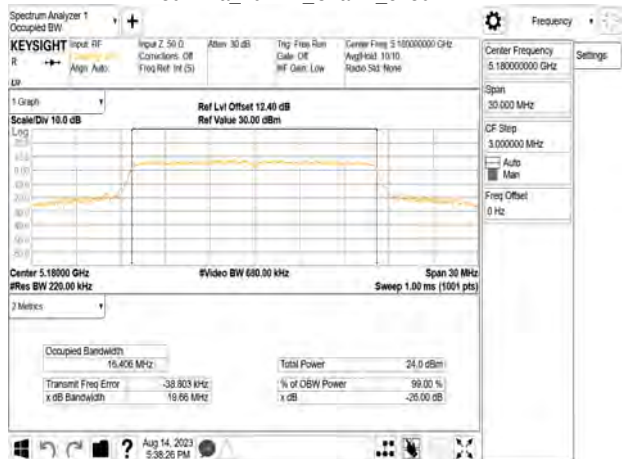
802.11a_20MHz_Chain2_5180MHz
