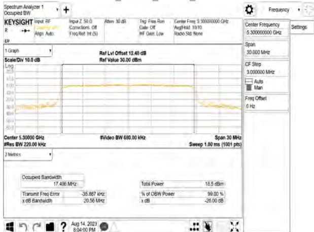
802.11n_20MHz_Chain0_5300MHz
