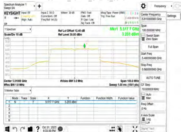
802.11n_40MHz_Chain3_5510MHz
