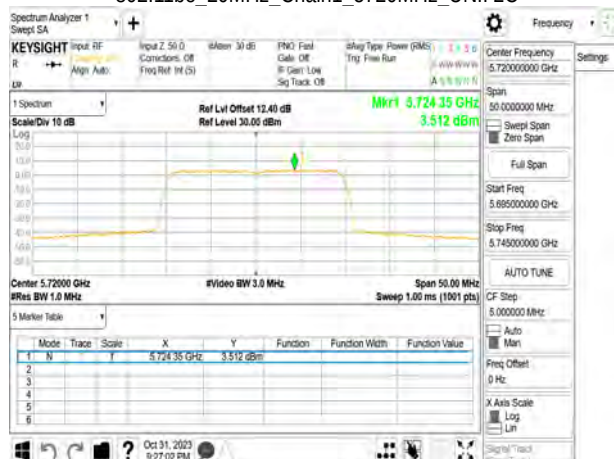
802.11be_20MHz_Chain1_5720MHz_UNII 2C
