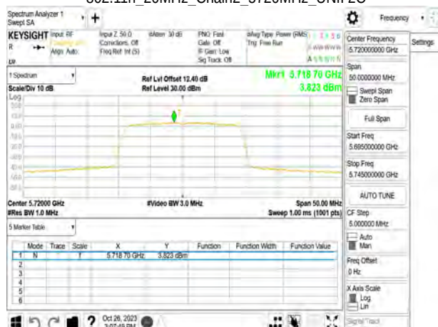
802.11n_20MHz_Chain2_5720MHz_UNII 3
