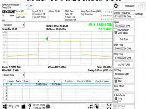
802.11be_40MHz_Chain3_5710MHz_UNII 3
