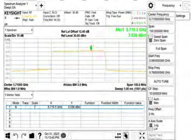
802.11be_40MHz_Chain0_5710MHz_UNII 3
