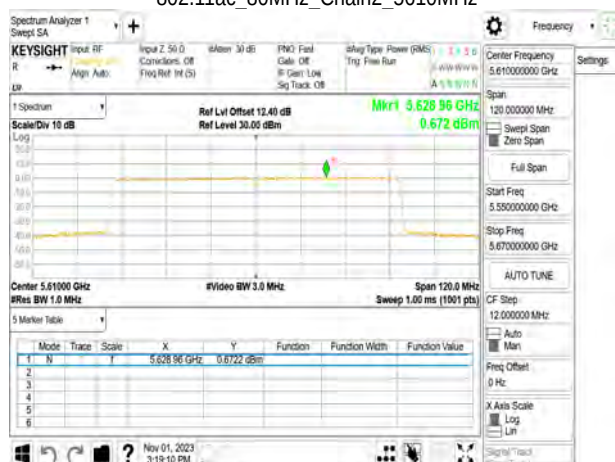
802.11ac_80MHz_Chain2_5610MHz
