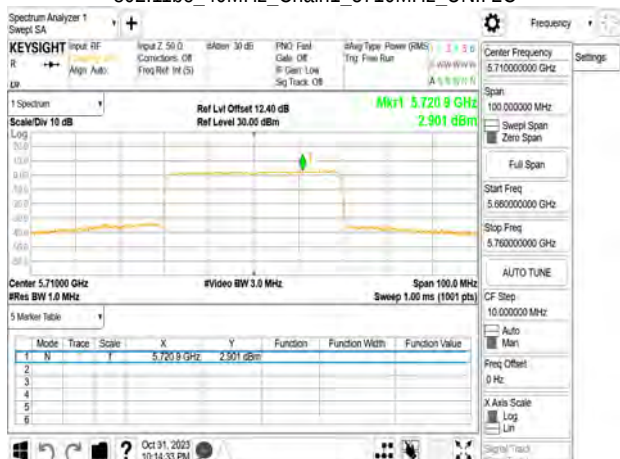
802.11be_40MHz_Chain1_5710MHz_UNII 2C
