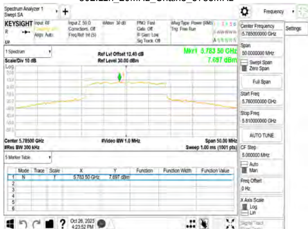
802.11n_20MHz_Chain3_5785MHz
