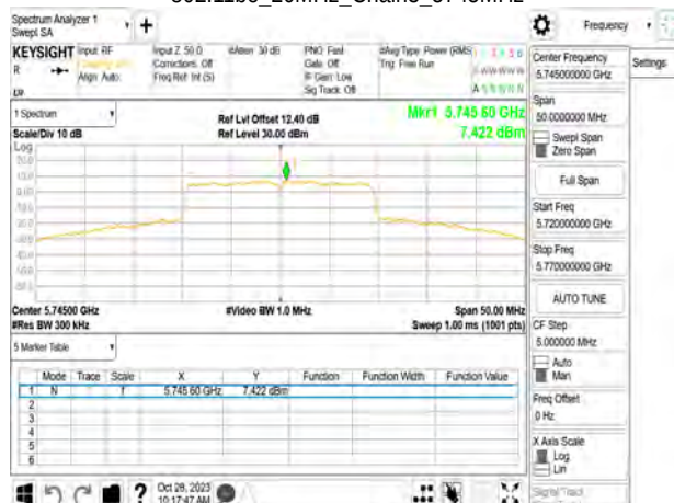
802.11be_20MHz_Chain3_5745MHz
