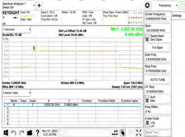
802.11ac_80MHz_Chain2_5690MHz_UNII 3
