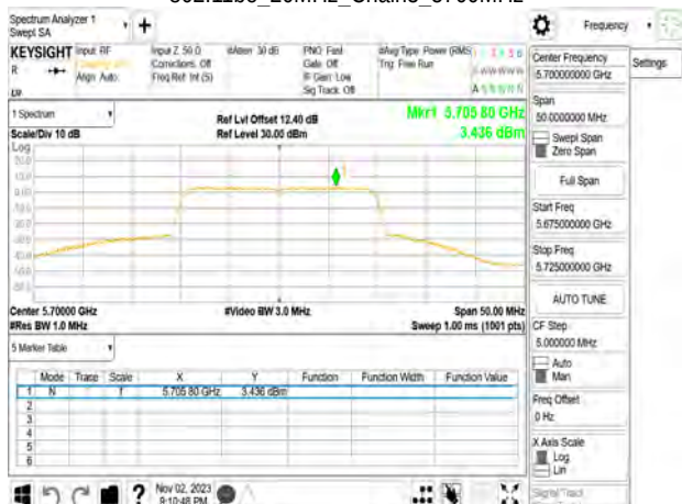
802.11be_20MHz_Chain3_5700MHz
