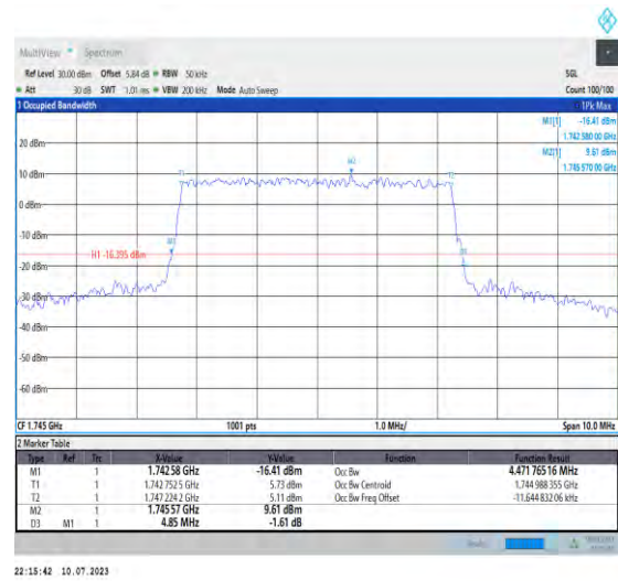
1-N66-PC3-15-5-M-6-CP-QPSK-Outer_Full-25@0-A nt3-4.472-4.850-≤5-PASS
