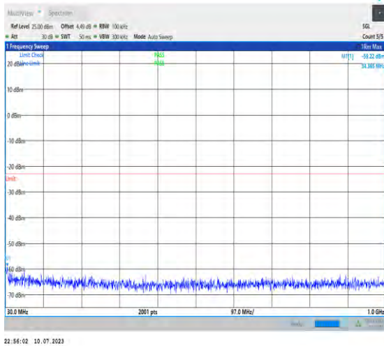
1-N66-PC3-15-40-M-1-DFT-PI2BPSK-Inner_1RB_L eft-1@1-30-1000-Ant3-34.37--59.22--23-PASS
