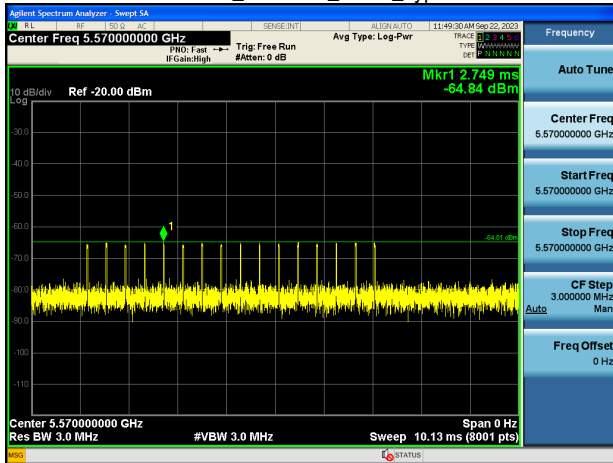
EHT160_5570MHz_Radar_Type 5
