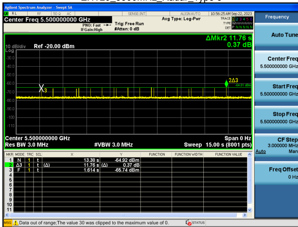
EHT20_5500MHz_Radar_Type 6
