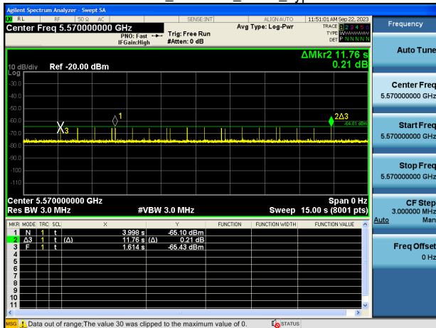
EHT160_5570MHz_Radar_Type 5
