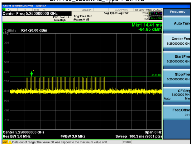
EHT160_5250MHz_Type 1-B.PNG
