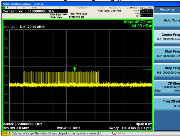
EHT40_5510MHz_Radar_Type 2
