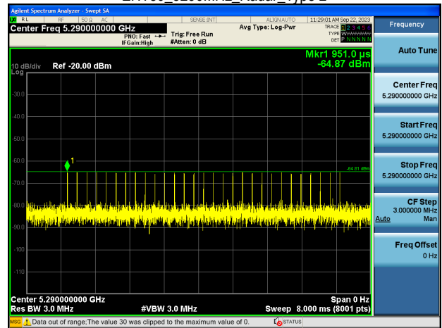
EHT80_5290MHz_Radar_Type 3
