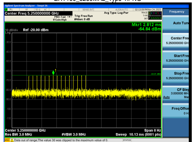
EHT160_5250MHz_Type 4.PNG
