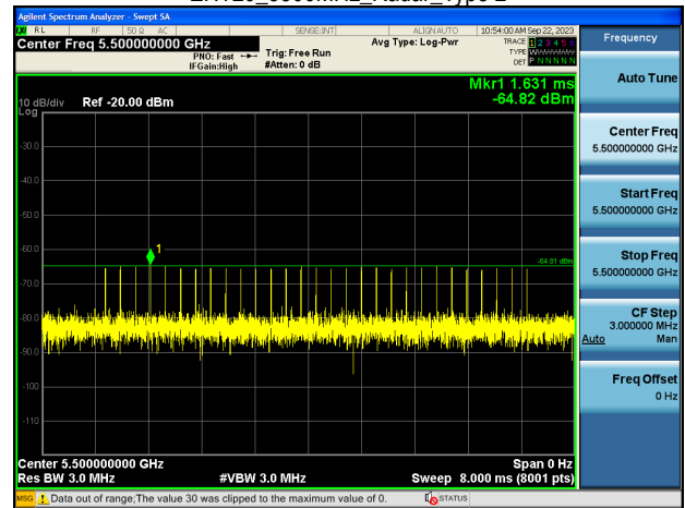
EHT20_5500MHz_Radar_Type 3
