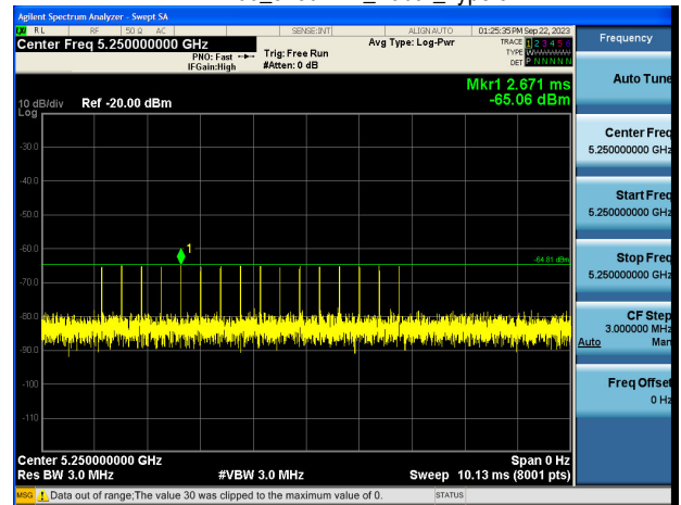
EHT160_5250MHz_Radar_Type 4
