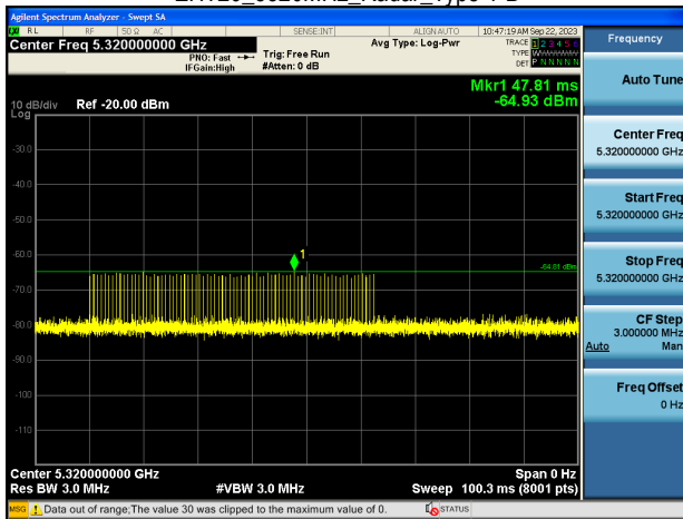
EHT20_5320MHz_Radar_Type 2
