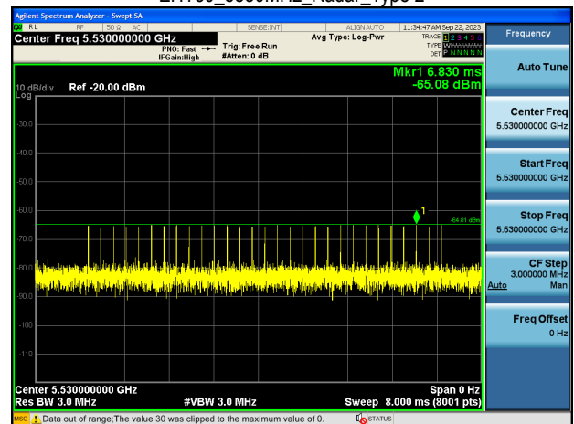
EHT80_5530MHz_Radar_Type 2
