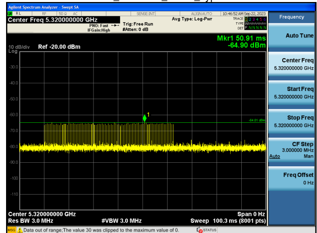
EHT20_5320MHz_Radar_Type 1-A
