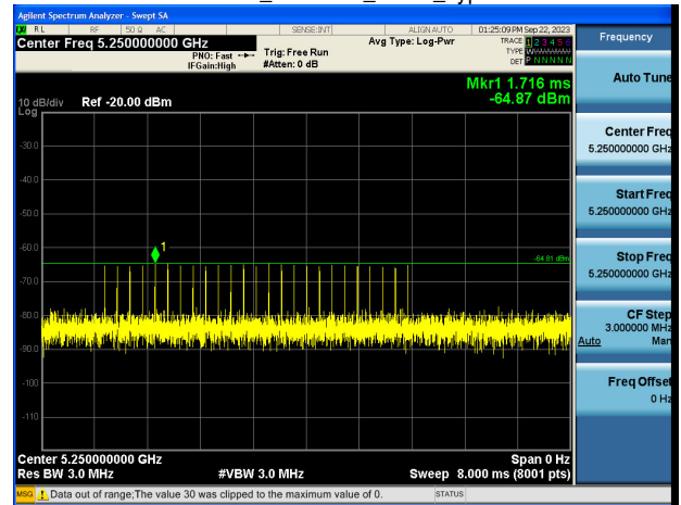
EHT160_5250MHz_Radar_Type 3
