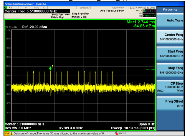
EHT40_5510MHz_Radar_Type 5
