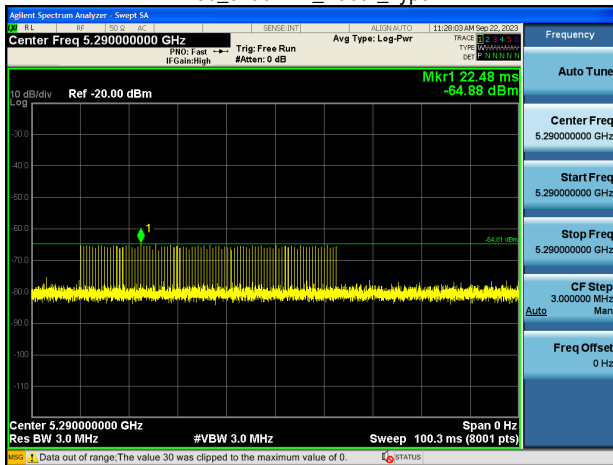
EHT80_5290MHz_Radar_Type 1-B
