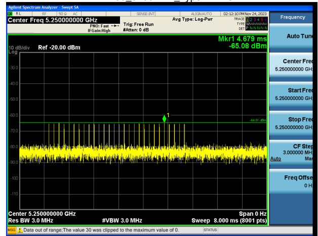
EHT160_5250MHz_Type 3.PNG
