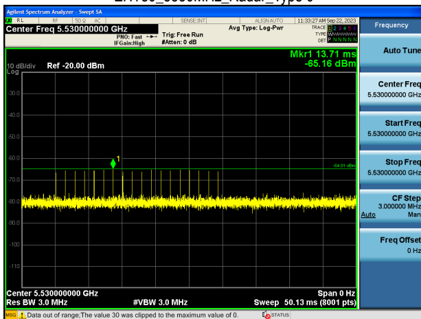
EHT80_5530MHz_Radar_Type 0
