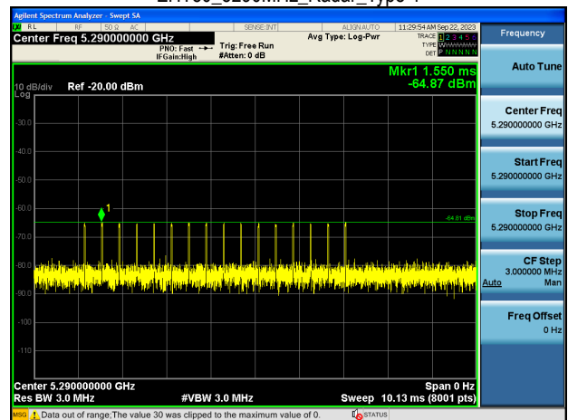
EHT80_5290MHz_Radar_Type 4
