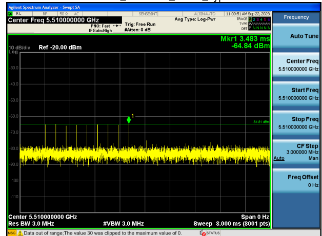
EHT40_5510MHz_Radar_Type 6
