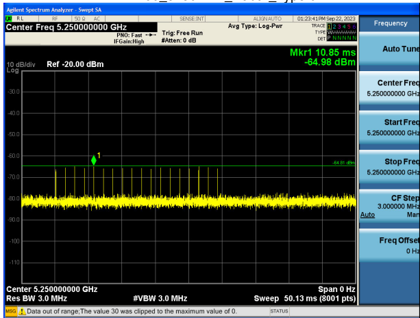
EHT160_5250MHz_Radar_Type 1-A
