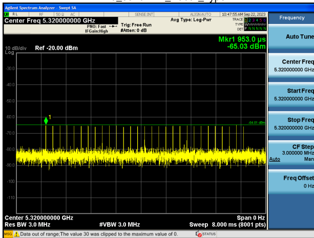
EHT20_5320MHz_Radar_Type 3
