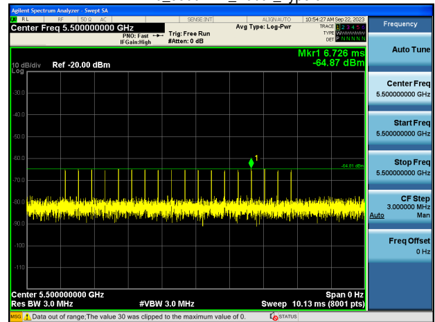
EHT20_5500MHz_Radar_Type 4
