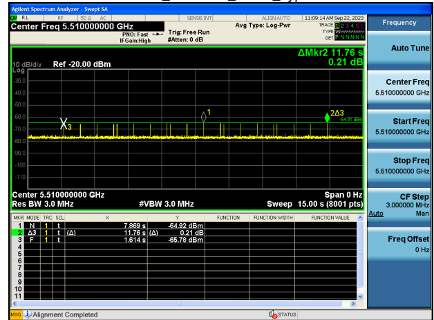
EHT40_5510MHz_Radar_Type 6
