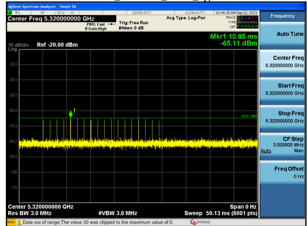
EHT20_5320MHz_Radar_Type 1-A
