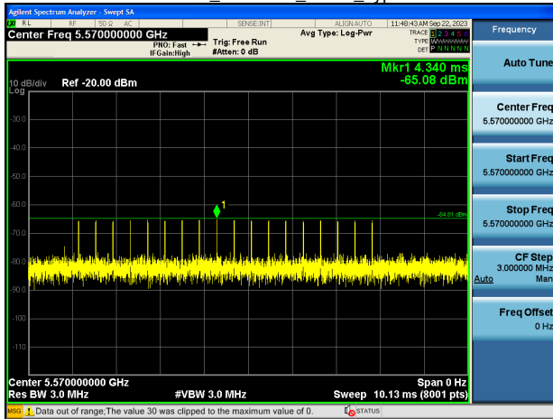
EHT160_5570MHz_Radar_Type 4
