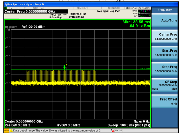
EHT80_5530MHz_Radar_Type 1-B
