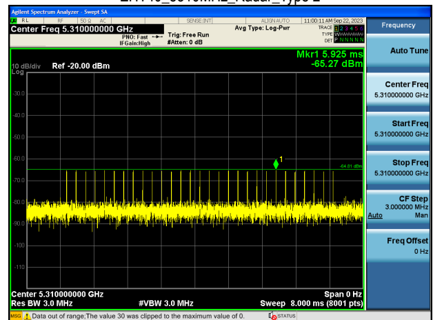
EHT40_5310MHz_Radar_Type 2
