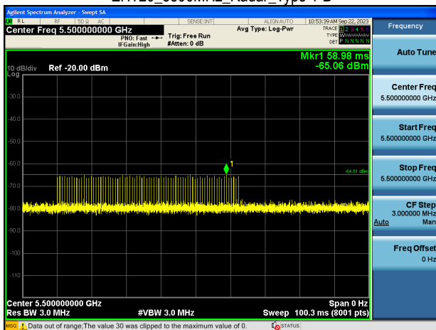
EHT20_5500MHz_Radar_Type 1-B
