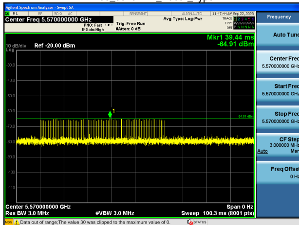
EHT160_5570MHz_Radar_Type 2
