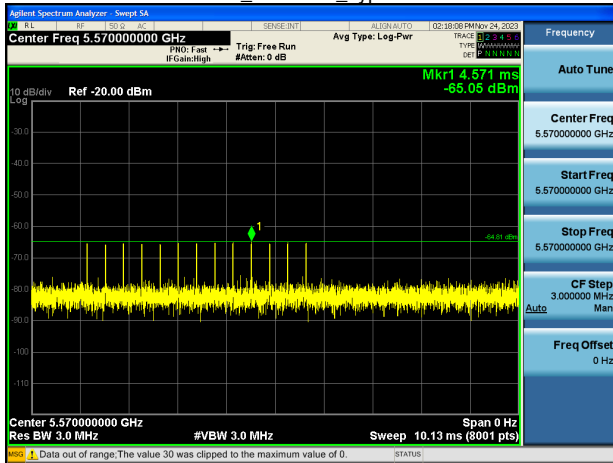
EHT160_5570MHz_Type 5.PNG
