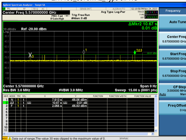
EHT160_5570MHz_Type 5.PNG
