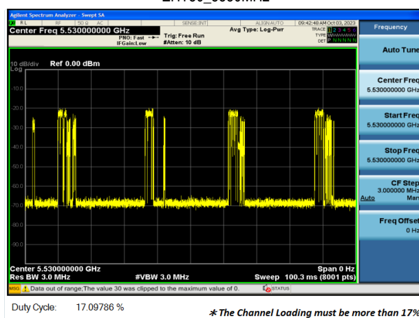
EHT80_5530MHz
