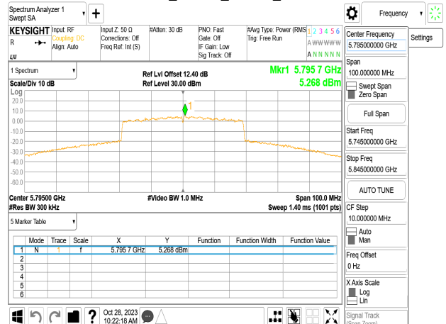
802.11be_40MHz_Chain1_5795MHz
