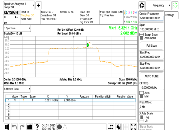
802.11be_40MHz_Chain0_5310MHz
