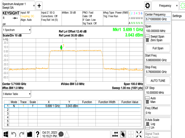
802.11be_40MHz_Chain2_5710MHz_UNII 3
