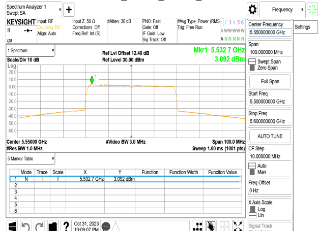
802.11be_40MHz_Chain2_5550MHz
