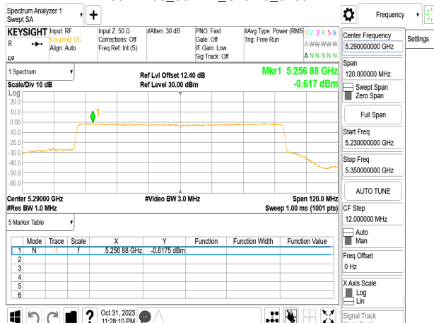
802.11be_80MHz_Chain0_5290MHz
