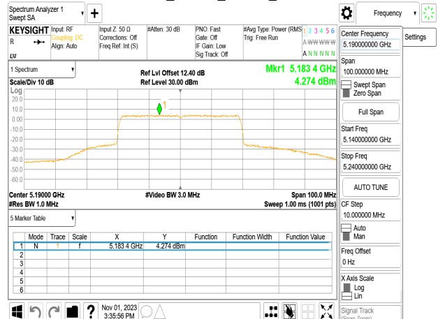
802.11be_40MHz_Chain3_5190MHz
