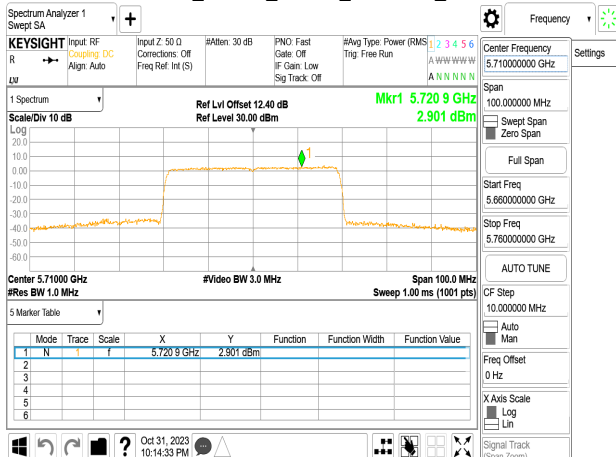
802.11be_40MHz_Chain1_5710MHz_UNII 2C
