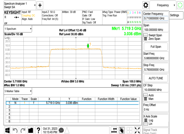
802.11be_40MHz_Chain0_5710MHz_UNII 3
