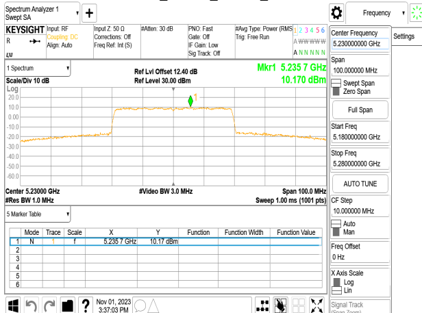
802.11be_40MHz_Chain1_5230MHz
