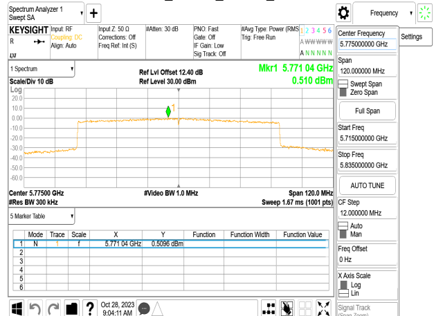
802.11be_80MHz_Chain1_5775MHz
