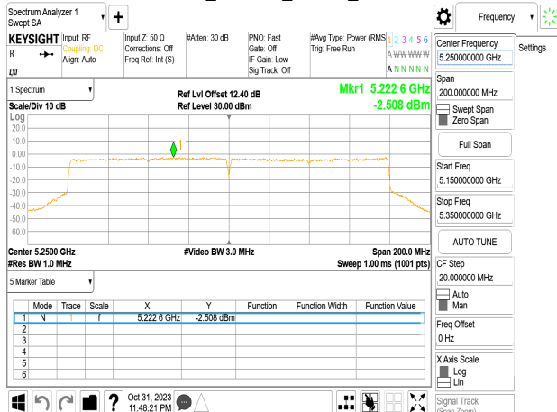
802.11be_160MHz_Chain0_5250MHz
