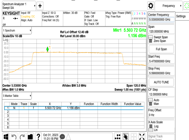
802.11be_80MHz_Chain2_5530MHz
