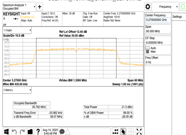
802.11n_40MHz_Chain1_5270MHz
