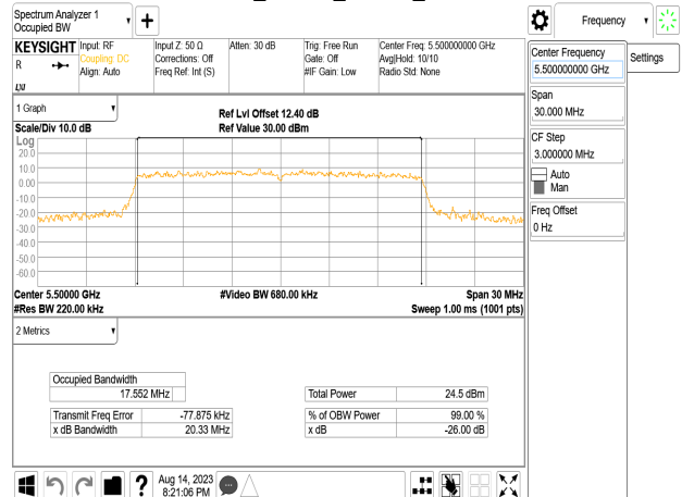
802.11n_20MHz_Chain1_5500MHz
