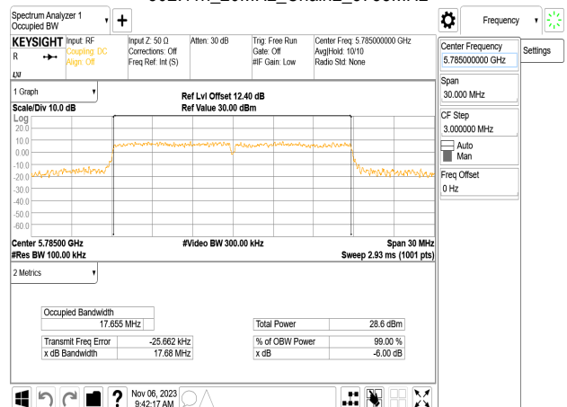
802.11n_20MHz_Chain2_5785MHz
