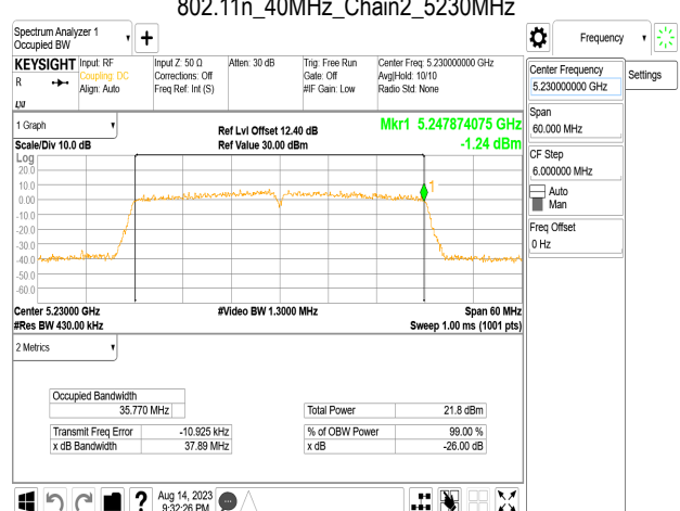
802.11n_40MHz_Chain2_5230MHz
