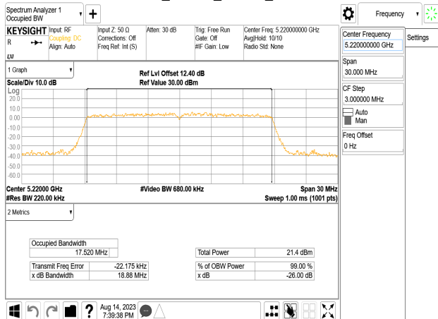
802.11n_20MHz_Chain3_5220MHz
