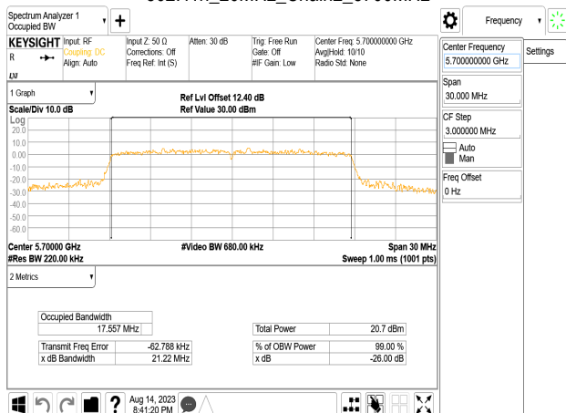
802.11n_20MHz_Chain2_5700MHz
