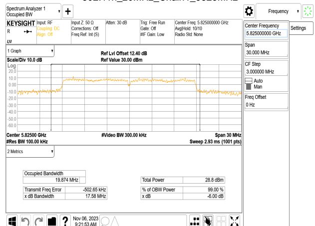
802.11n_20MHz_Chain1_5825MHz
