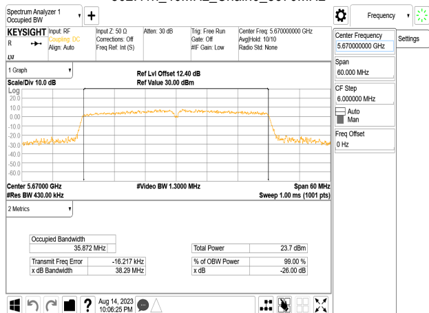
802.11n_40MHz_Chain0_5670MHz
