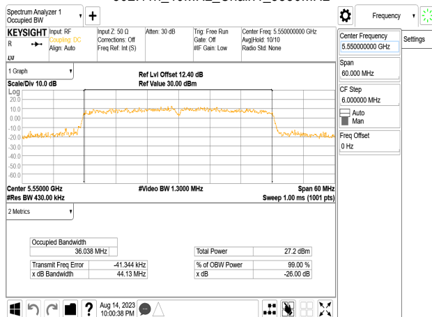
802.11n_40MHz_Chain1_5550MHz
