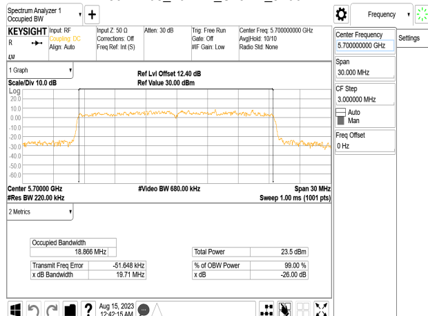
802.11be_20MHz_Chain1_5700MHz
