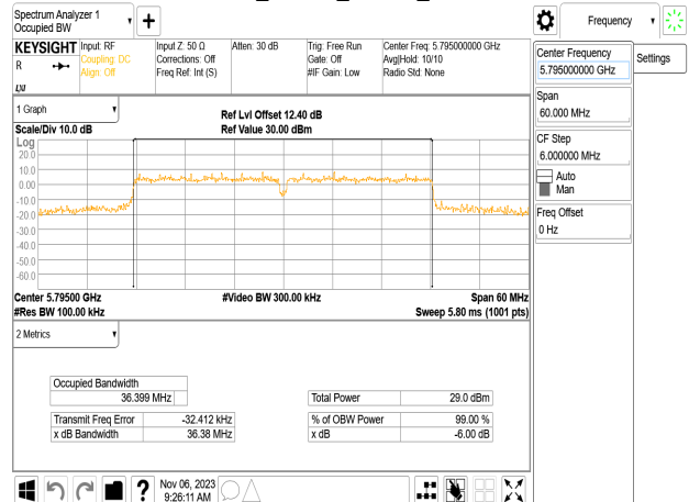
802.11n_40MHz_Chain3_5795MHz
