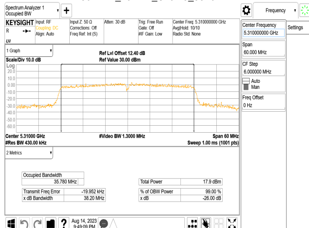
802.11n_40MHz_Chain3_5310MHz
