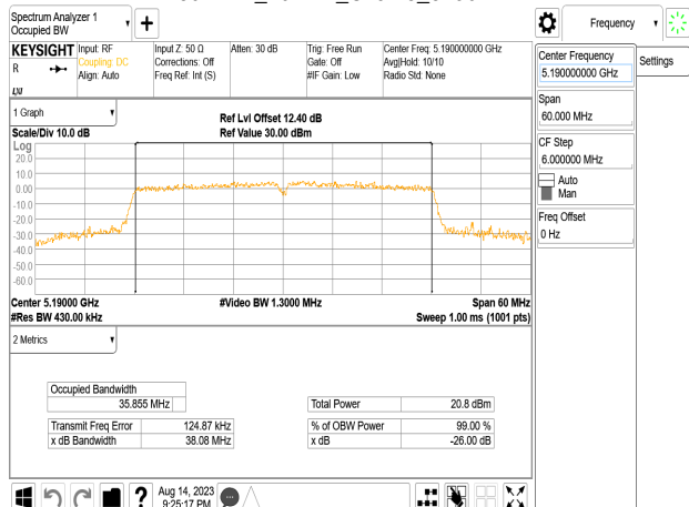
802.11n_40MHz_Chain3_5190MHz
