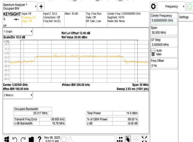
802.11be_20MHz_Chain0_5825MHz
