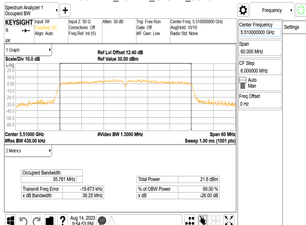
802.11n_40MHz_Chain2_5510MHz
