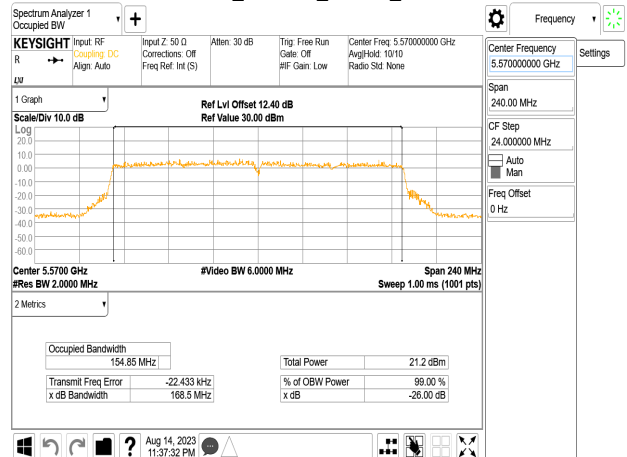
802.11ac_160MHz_Chain2_5570MHz
