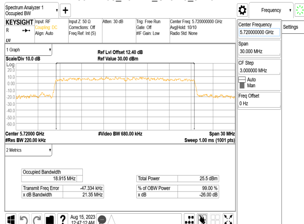
802.11be_20MHz_Chain0_5720MHz
