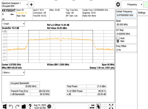
802.11n_40MHz_Chain3_5670MHz
