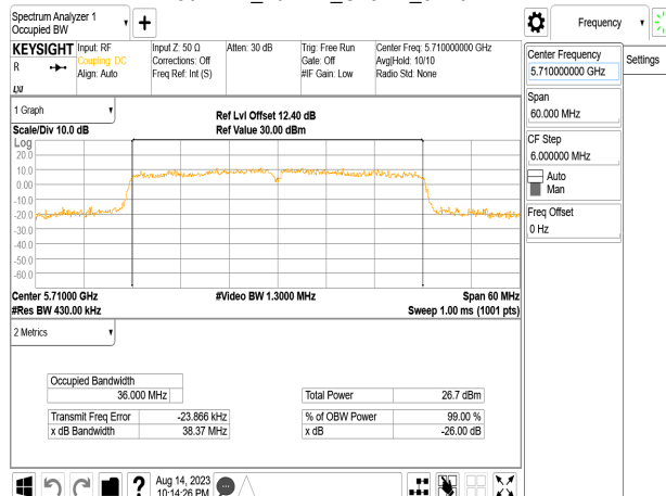
802.11n_40MHz_Chain2_5710MHz
