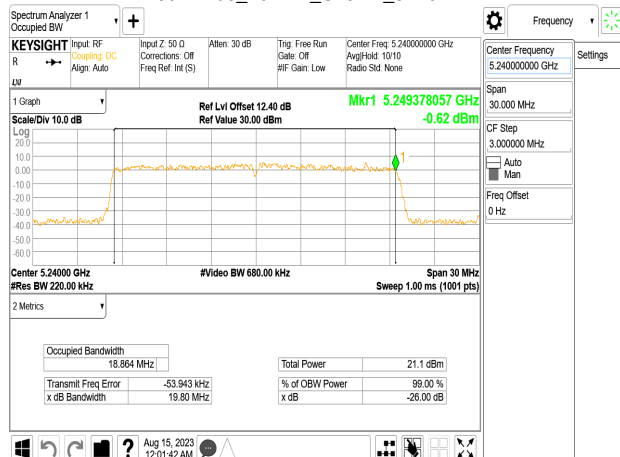
802.11be_20MHz_Chain1_5240MHz
