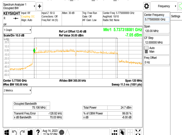
802.11ac_80MHz_Chain2_5775MHz
