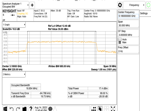
802.11be_20MHz_Chain0_5180MHz
