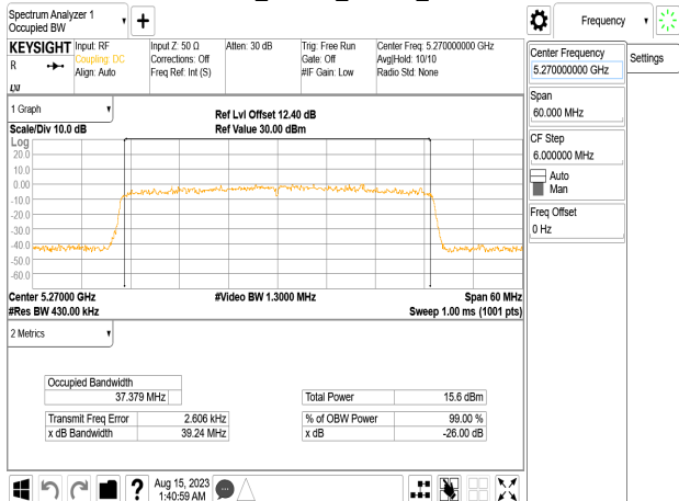
802.11be_40MHz_Chain0_5270MHz
