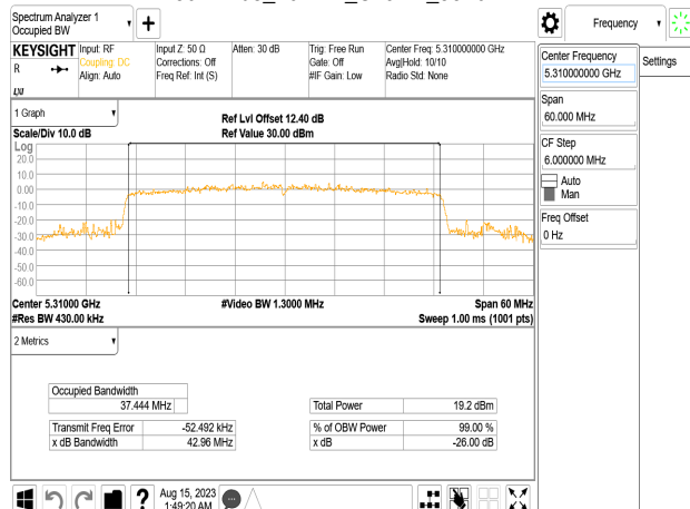
802.11be_40MHz_Chain2_5310MHz
