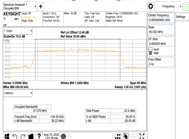
802.11be_40MHz_Chain3_5550MHz
