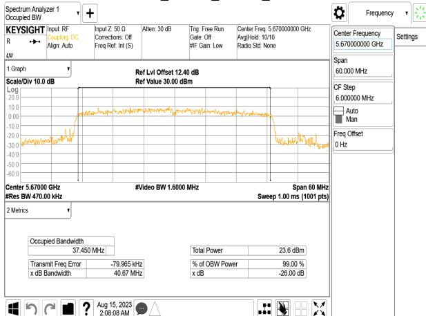
802.11be_40MHz_Chain2_5670MHz
