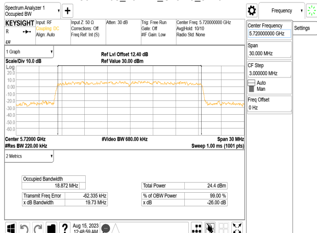
802.11be_20MHz_Chain3_5720MHz
