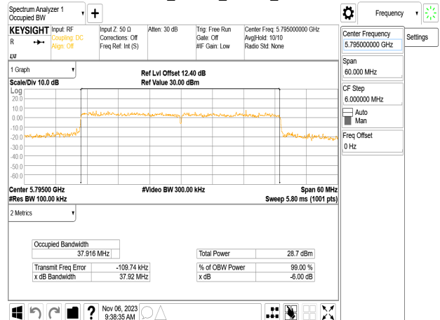
802.11be_40MHz_Chain2_5795MHz
