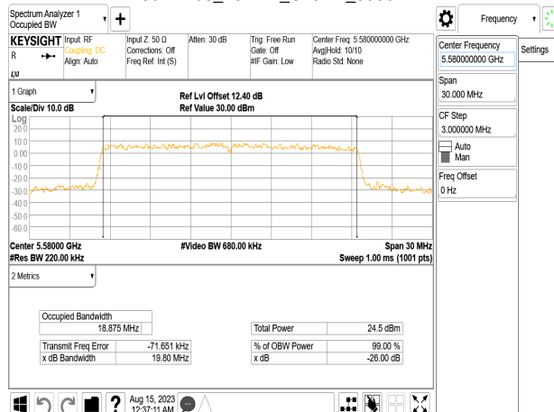
802.11be_20MHz_Chain2_5580MHz
