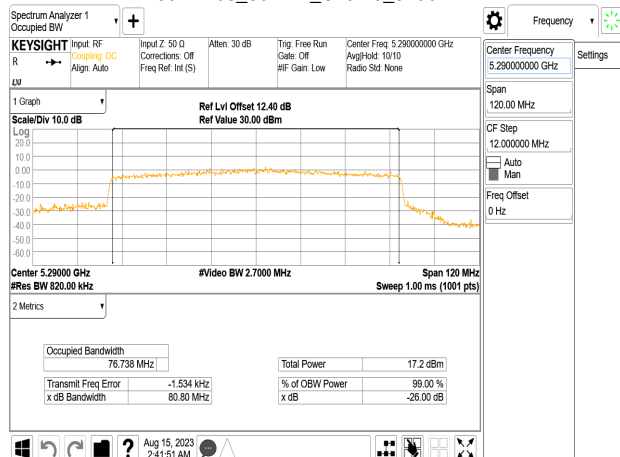
802.11be_80MHz_Chain0_5290MHz
