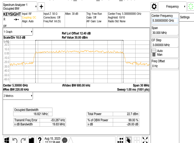
802.11be_20MHz_Chain2_5300MHz
