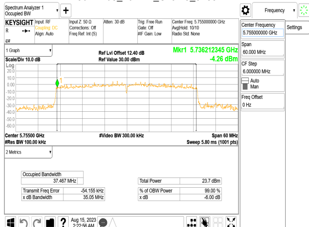
802.11be_40MHz_Chain3_5755MHz
