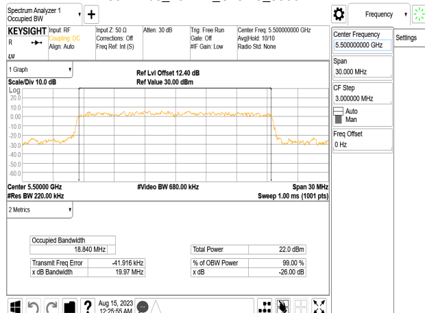
802.11be_20MHz_Chain3_5500MHz
