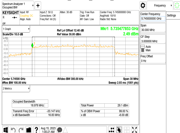
802.11be_20MHz_Chain2_5745MHz
