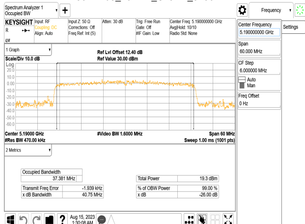
802.11be_40MHz_Chain2_5190MHz
