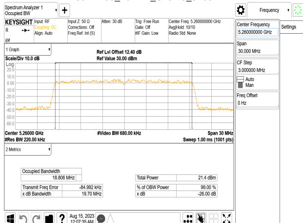
802.11be_20MHz_Chain3_5260MHz
