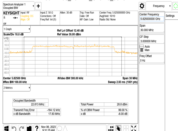
802.11be_20MHz_Chain3_5825MHz
