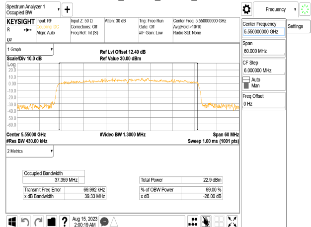
802.11be_40MHz_Chain0_5550MHz
