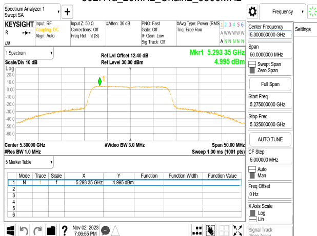
802.11a_20MHz_Chain2_5300MHz
