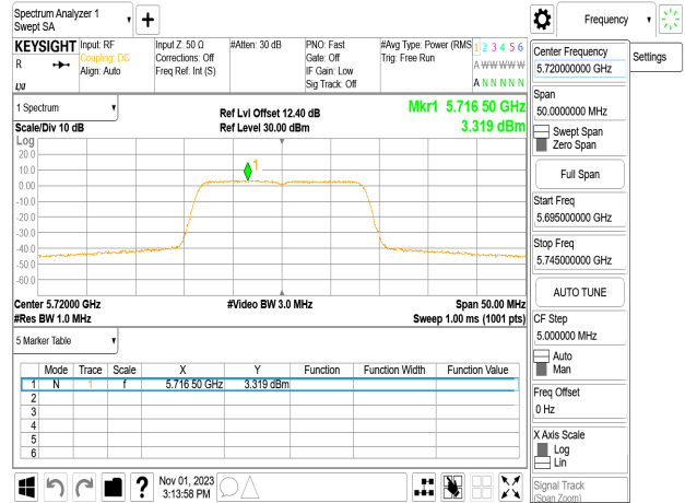
802.11a_20MHz_Chain3_5720MHz_UNII 3
