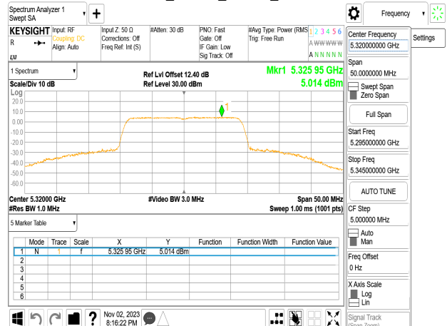
802.11n_20MHz_Chain2_5320MHz
