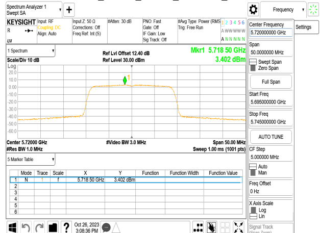
802.11n_20MHz_Chain3_5720MHz_UNII 2C
