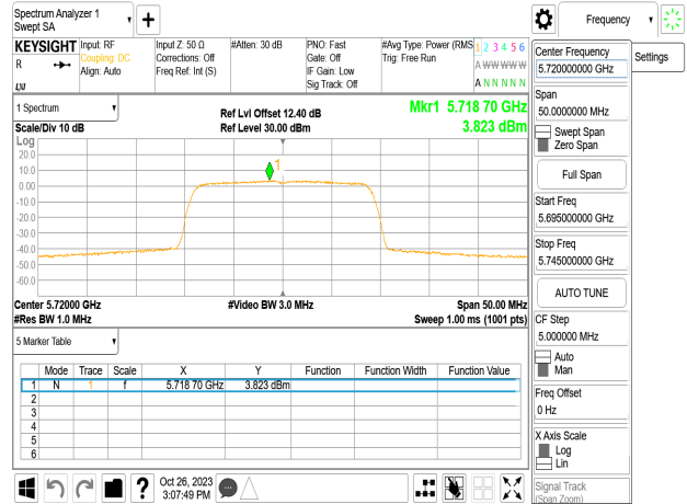
802.11n_20MHz_Chain2_5720MHz_UNII 3
